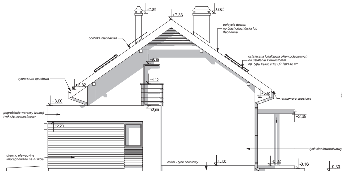
ELEWACJA BOCZNA
