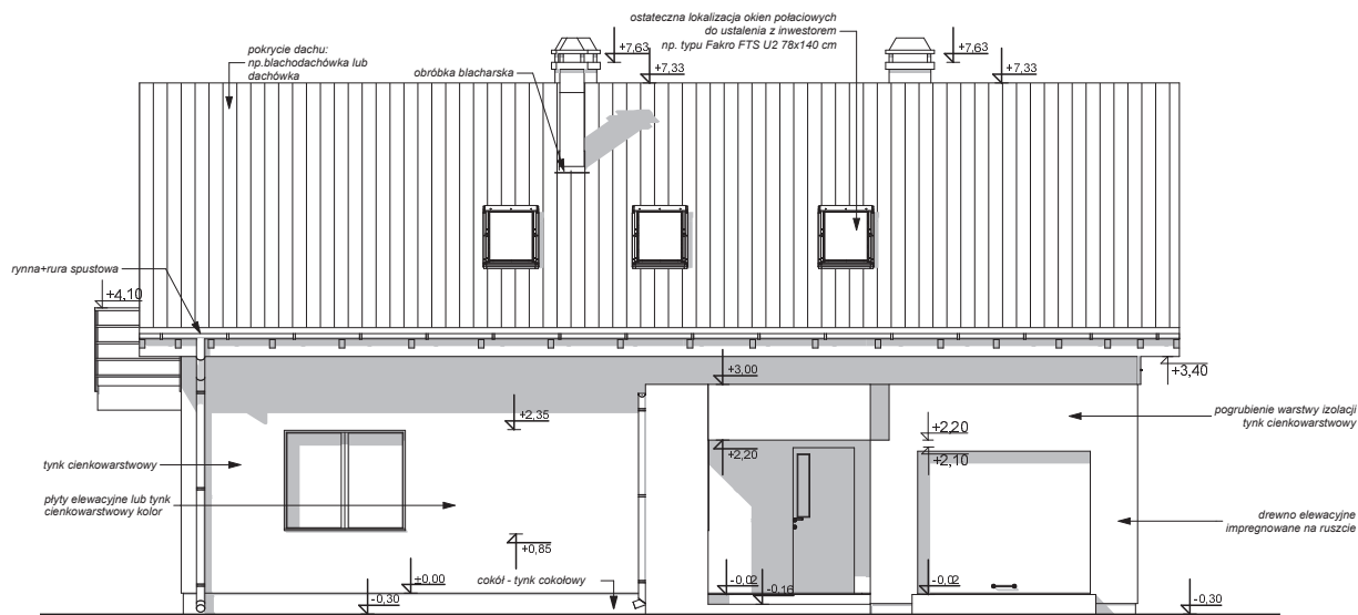
ELEWACJA FRONTOWA
