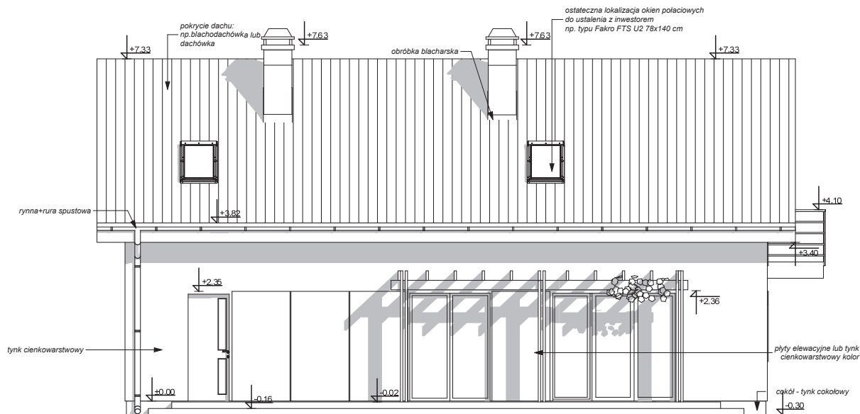
ELEWACJA TYLNA
