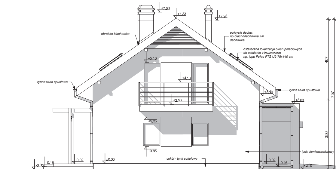
ELEWACJA BOCZNA
