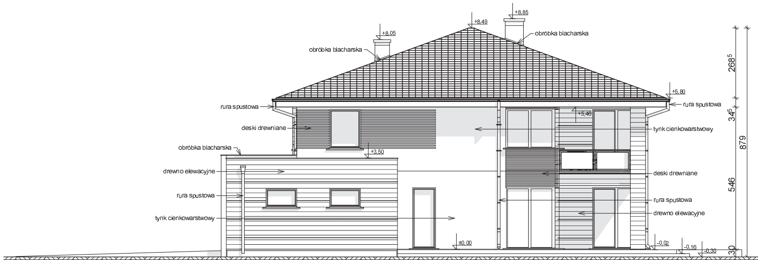
ELEWACJA BOCZNA
