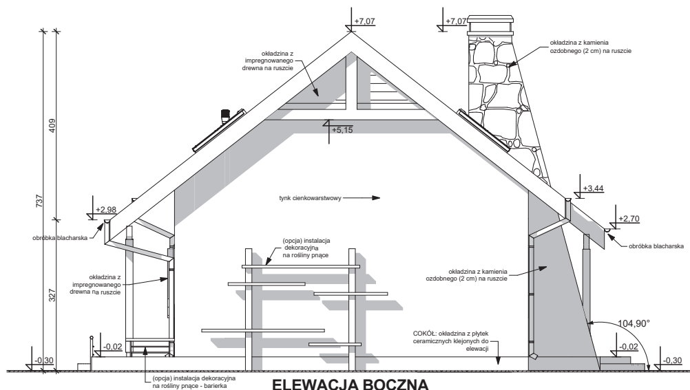
ELEWACJA BOCZNA
