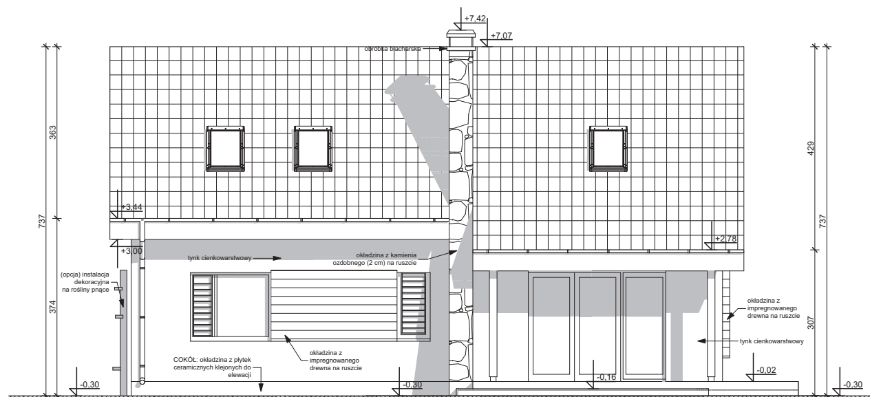
ELEVACJA OGRODOWA
