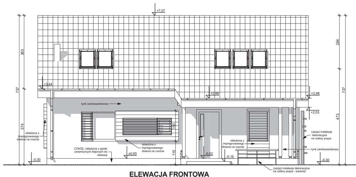
ELEWACJA FRONTOWA
