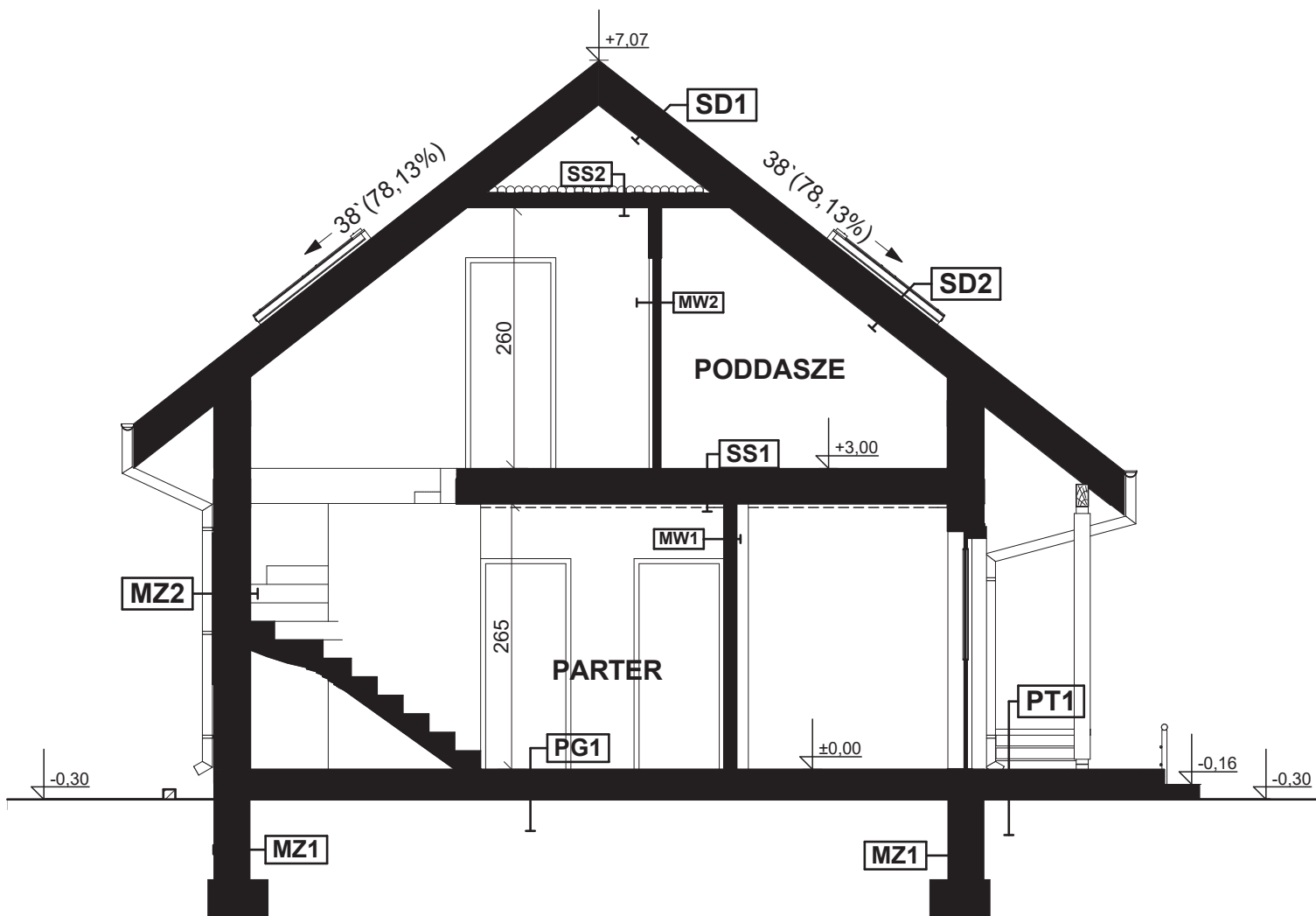
PRZEKRÓJ A-A
