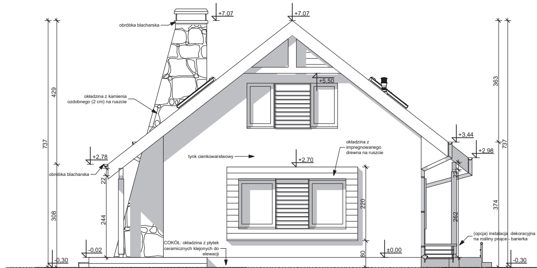
ELEVACJA BOCZNA
