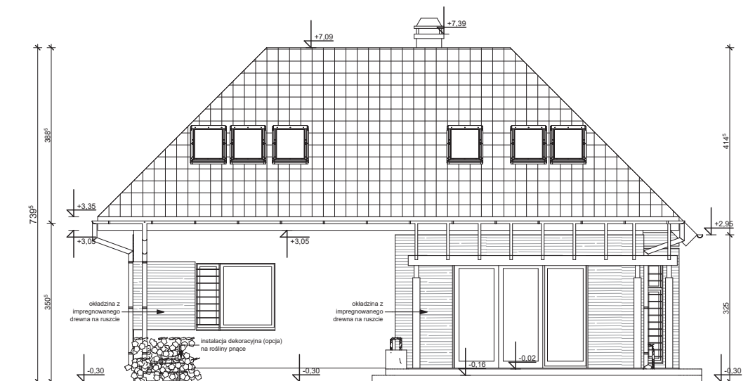
ELEWACJA TYLNA
