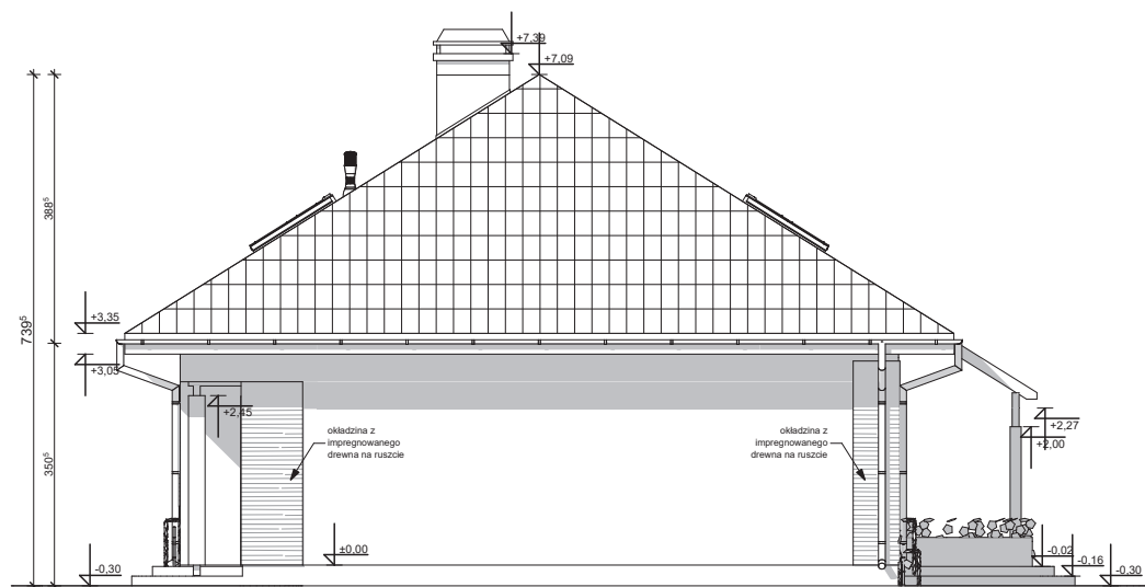
ELEWACJA BOCZNA
