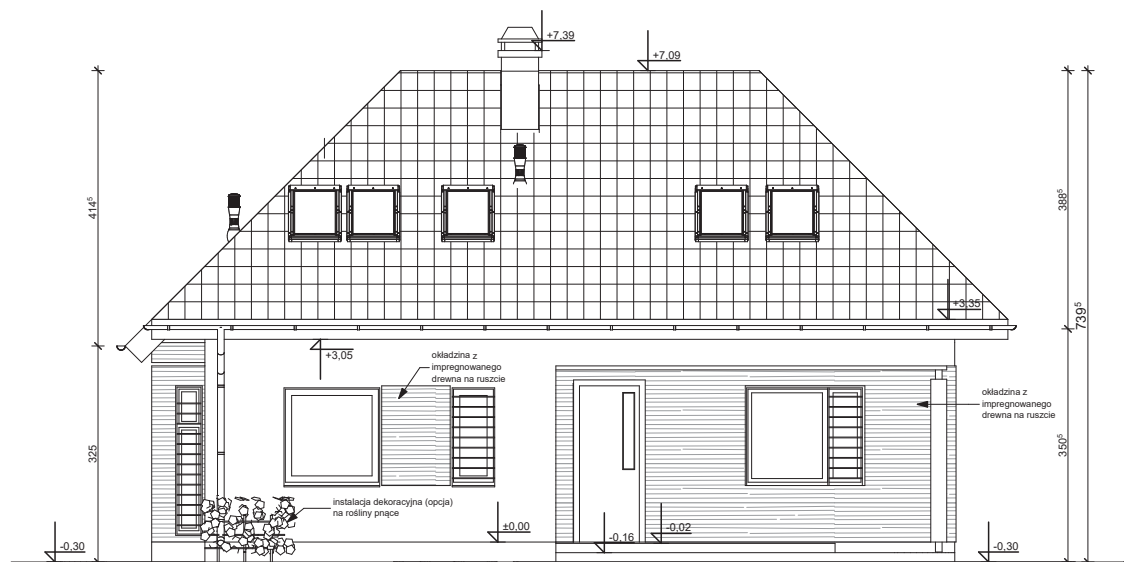
ELEWACJA FRONTOWA
