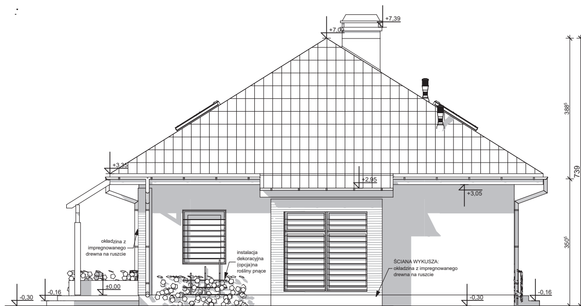
ELEWACJA BOCZNA
