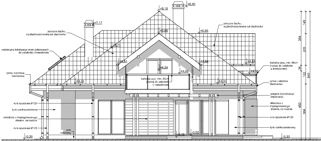
ELEWACJA OGRODOWA
