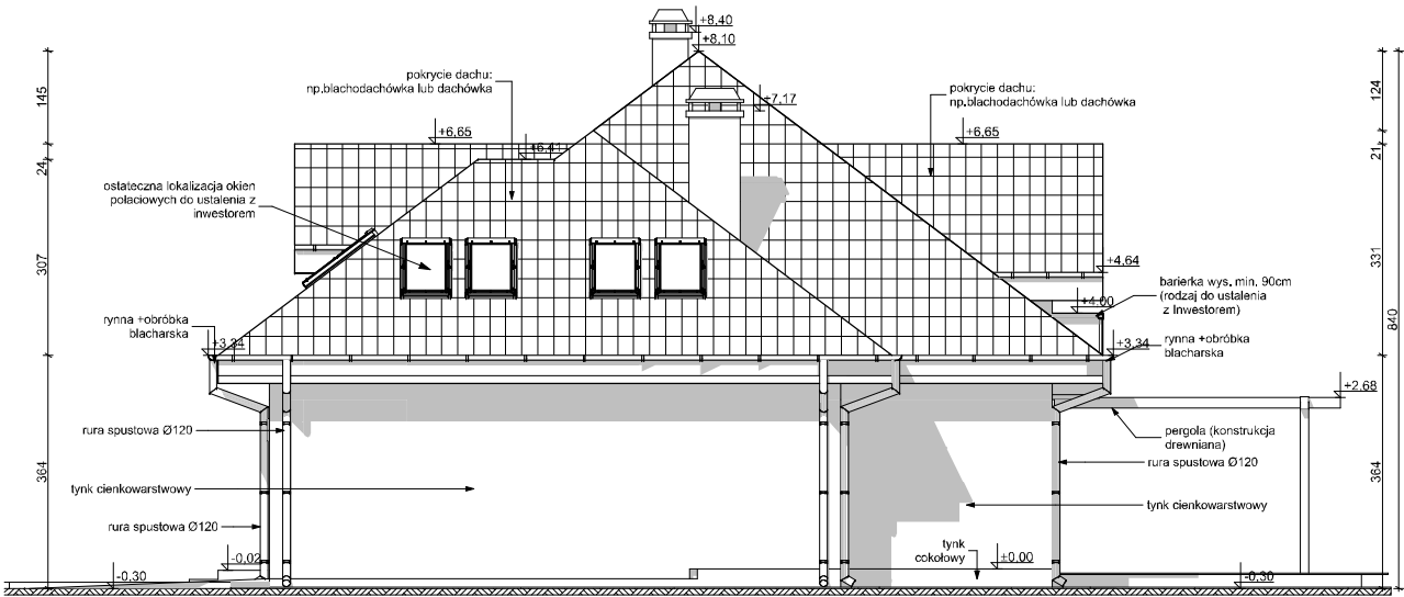
ELEWACJA BOCZNA
