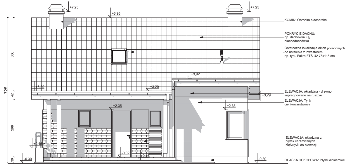
ELEWACJA FRONTOWA
