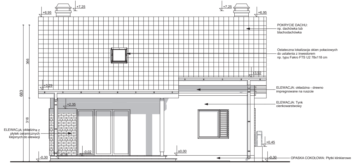
ELEWACJA OGRODOWA
