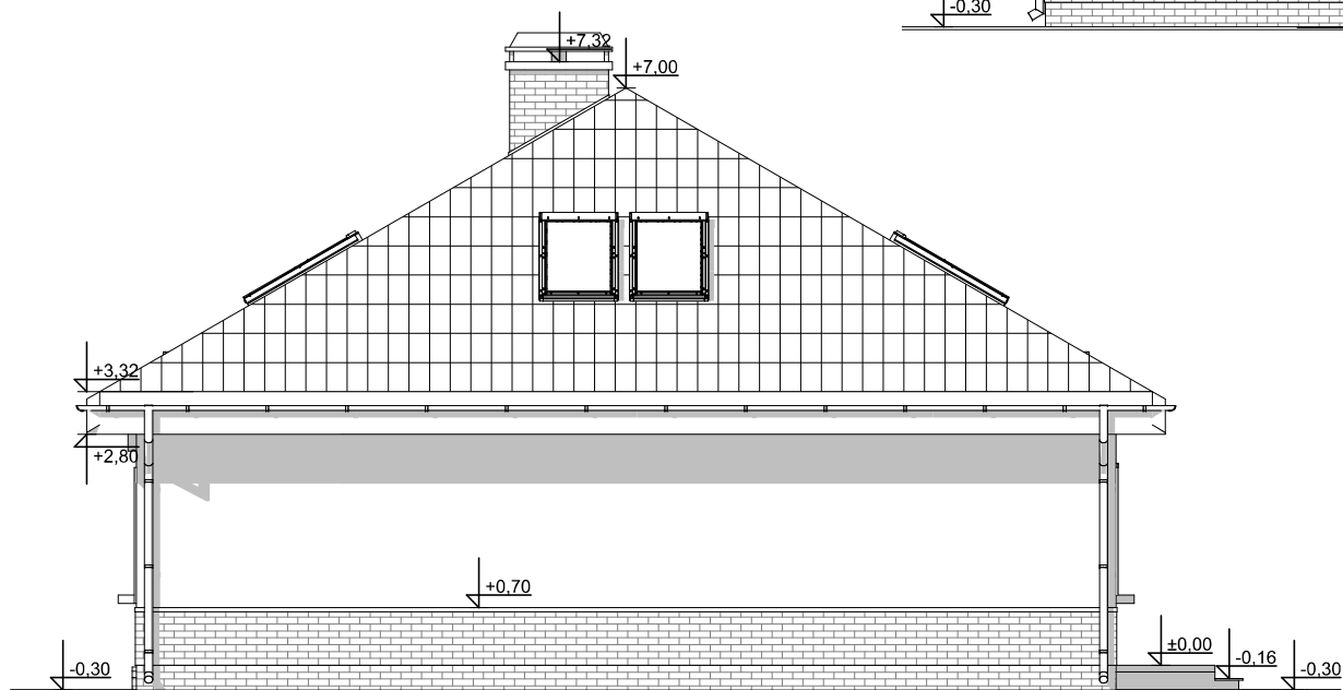
ELEWACJA BOCZNA
