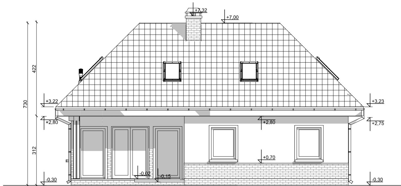
ELEWACJA OGRODOWA
