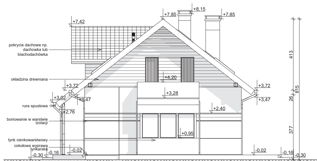
ELEWACJA BOCZNA
