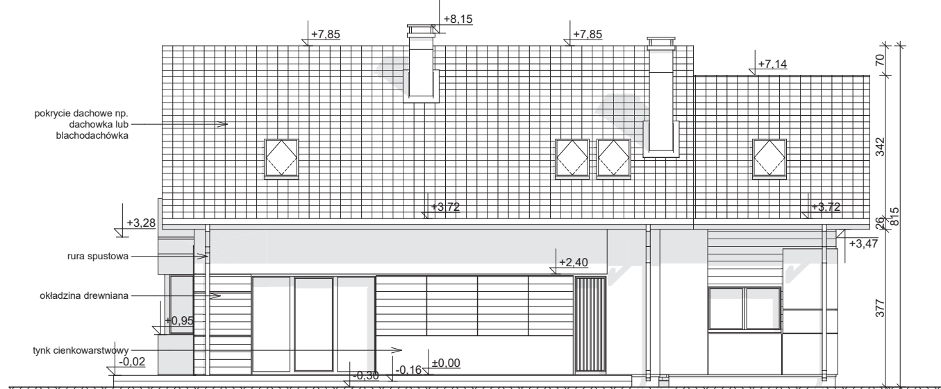
ELEWACJA TYLNA
