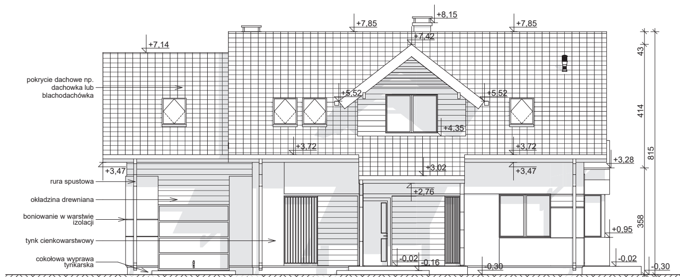
ELEWACJA FRONTOWA
