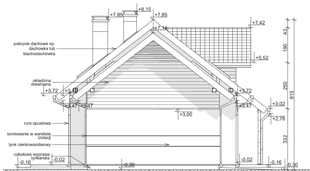
ELEWACJA BOCZNA
