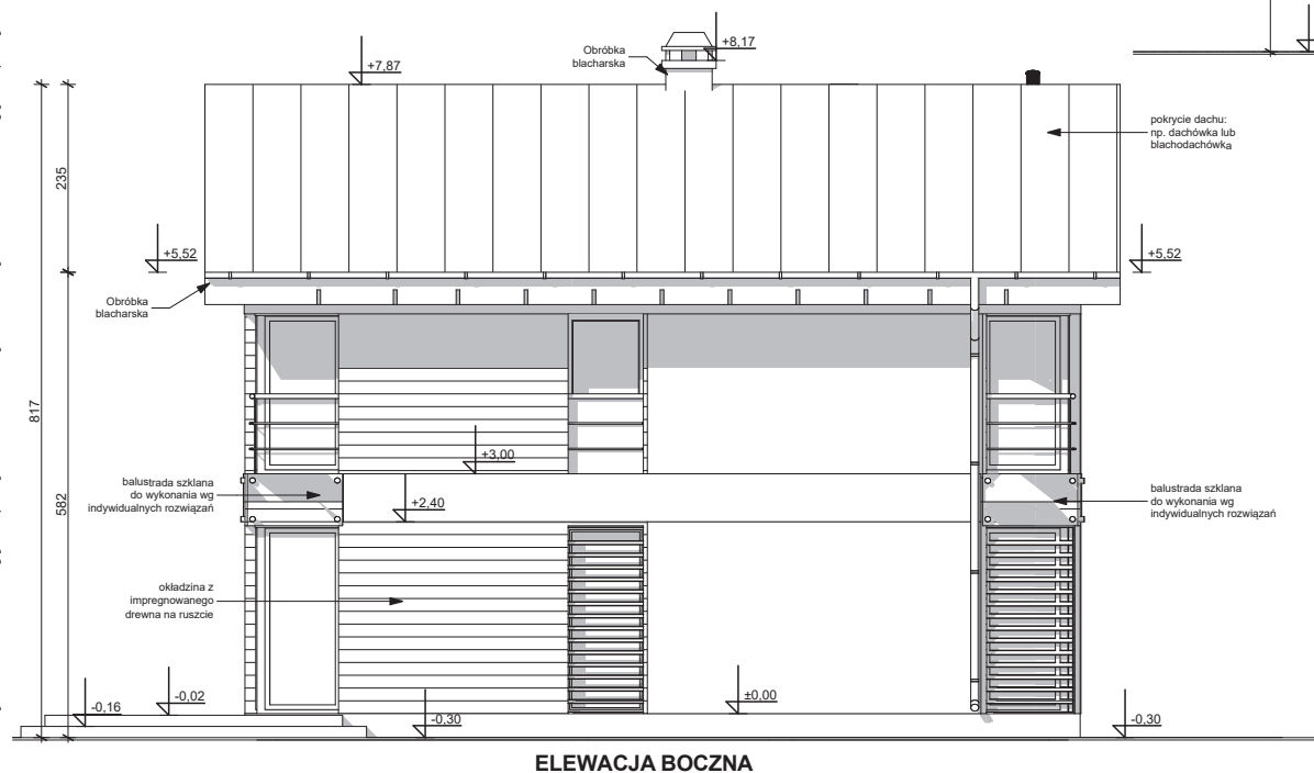
ELEWACJA BOCZNA
