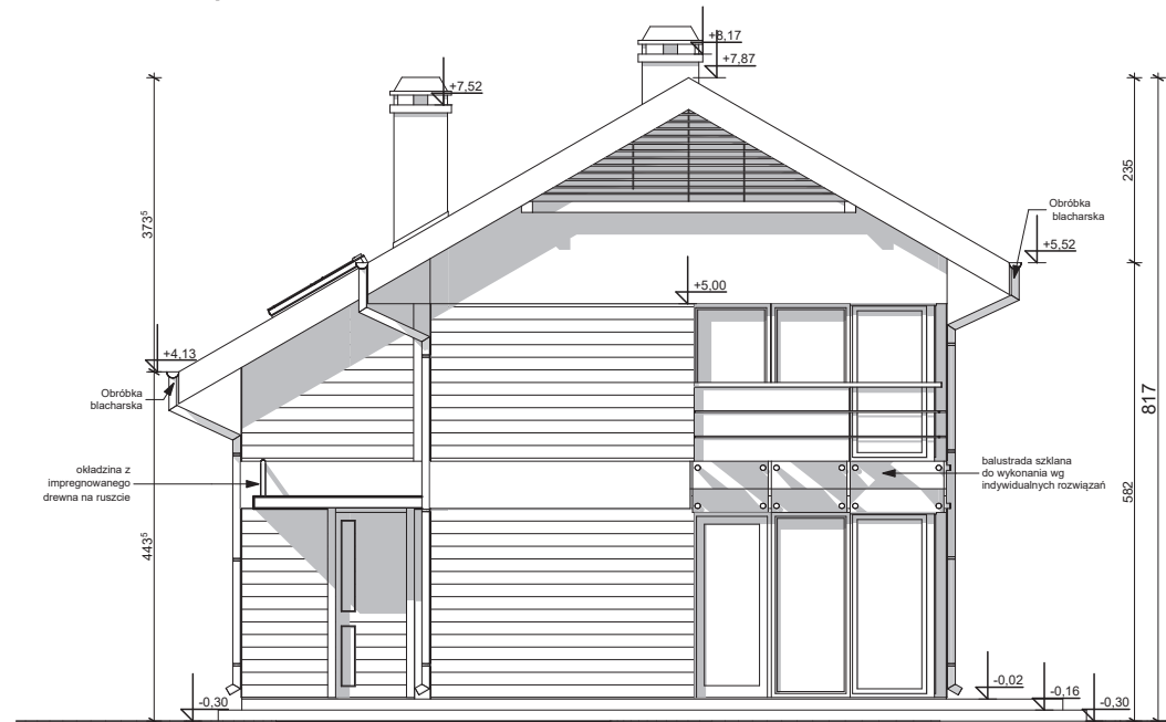
ELEWACJA FRONTOWA
