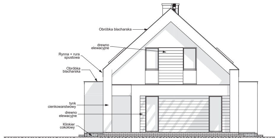
ELEWACJA OGRODOWA
