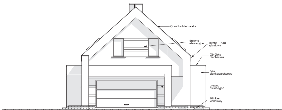
ELEWACJA FRONTOWA
