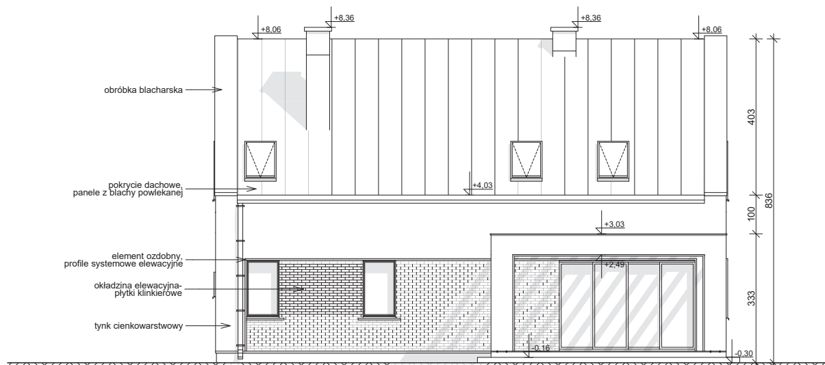
ELEWACJA OGRODOWA
