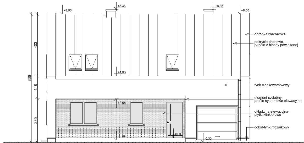
ELEWACJA FRONTOWA
