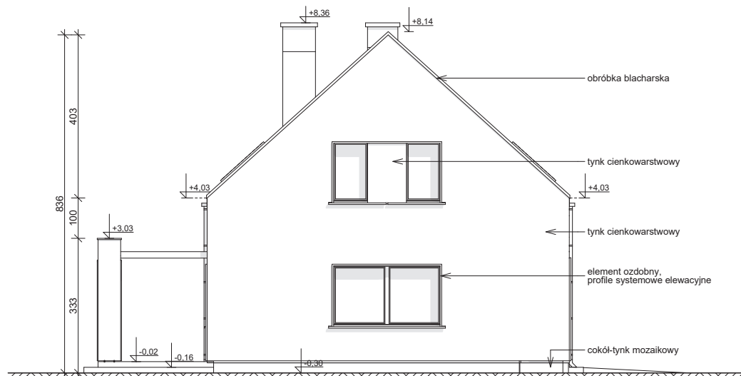
ELEWACJA BOCZNA
