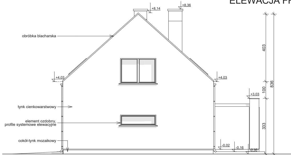
ELEWACJA BOCZNA
