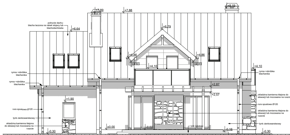
ELEWACJA OGRODOWA
