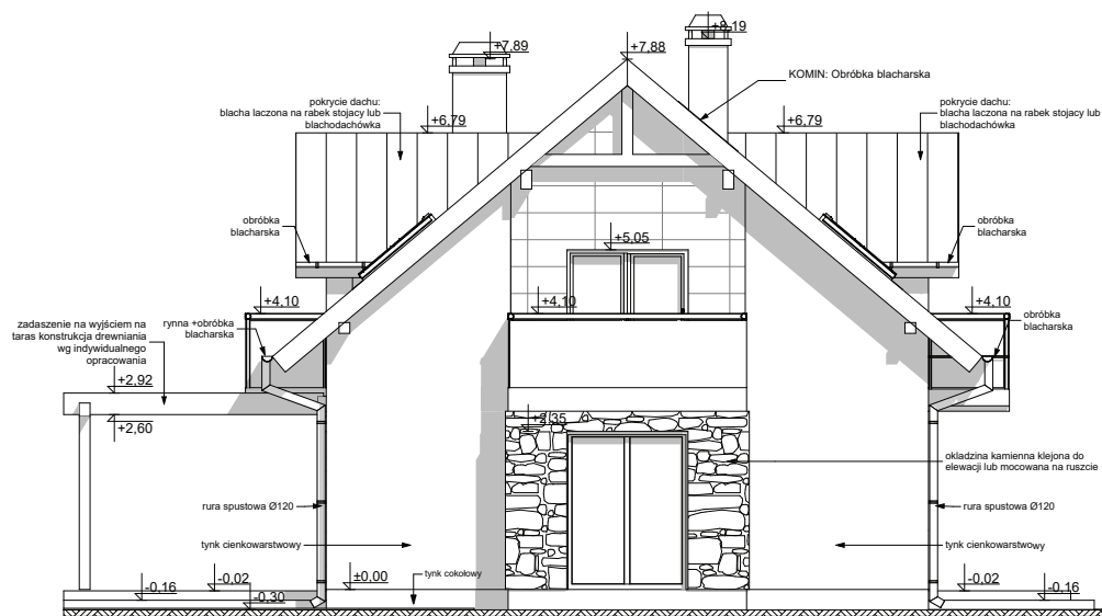
ELEWACJA BOCZNA
