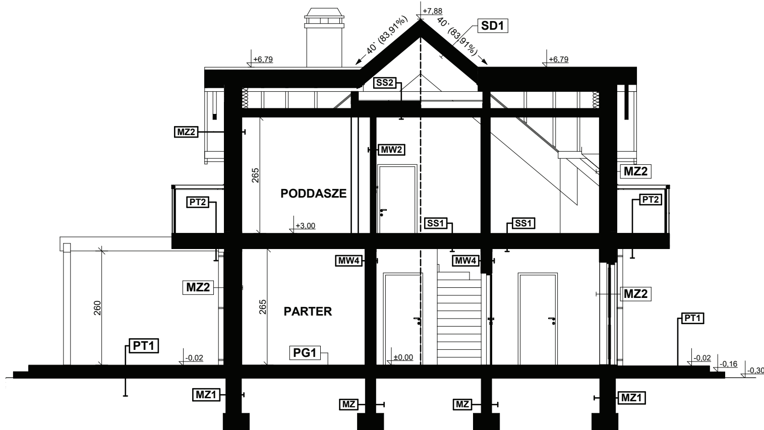
PRZEKRÓJ B-B
