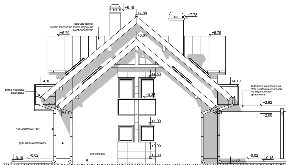
ELEWACJA BOCZNA
