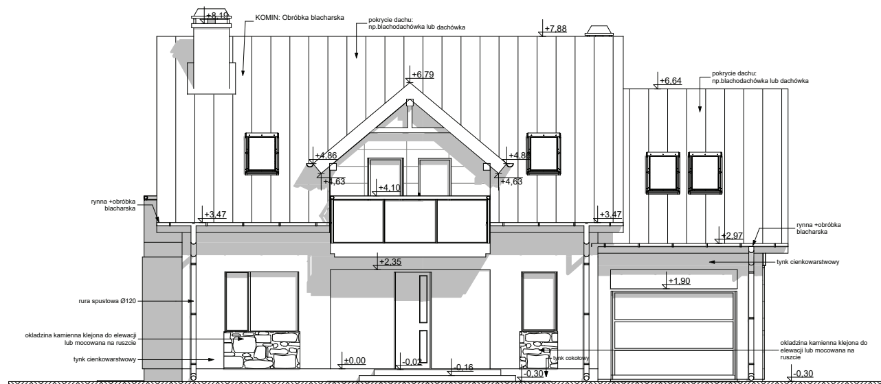
ELEWACJA FRONTOWA
