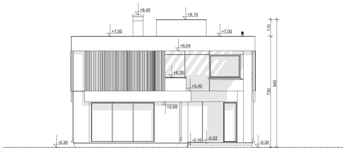
ELEWACJA OGRODOWA
