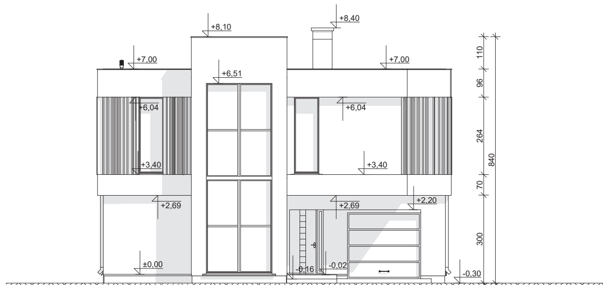
ELEWACJA FRONTOWA
