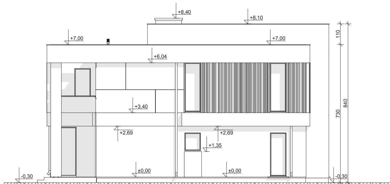
ELEWACJA BOCZNA
