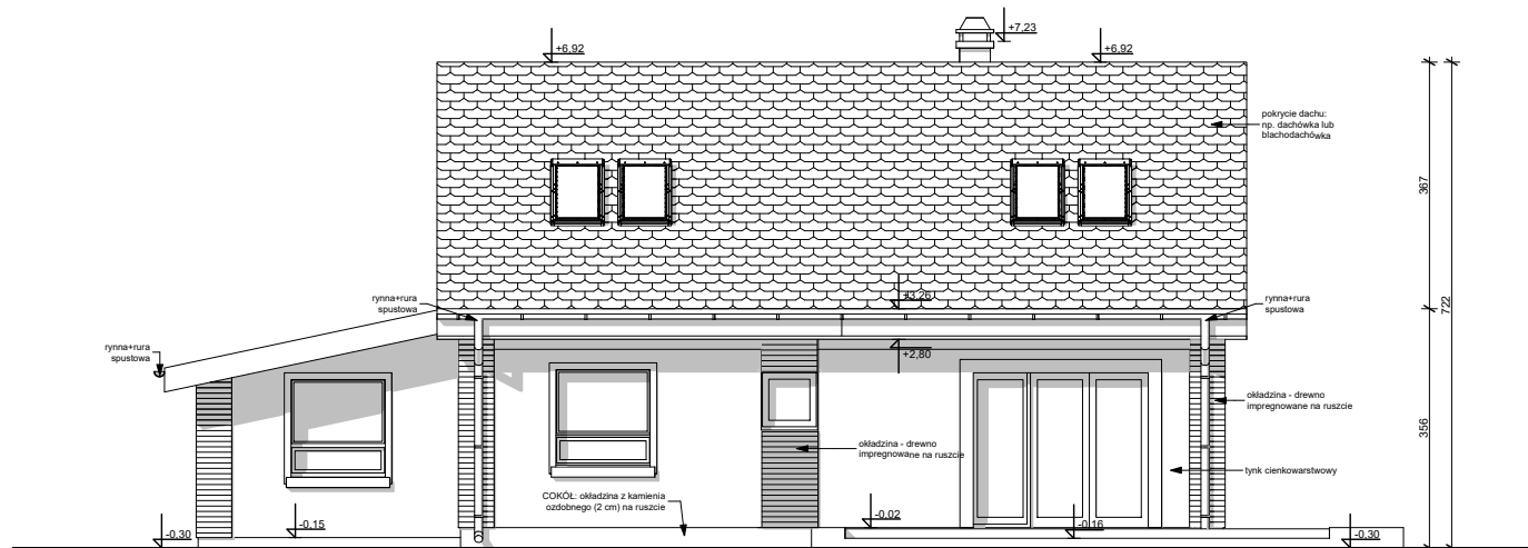
ELEWACJA OGRODOWA (tylna)
