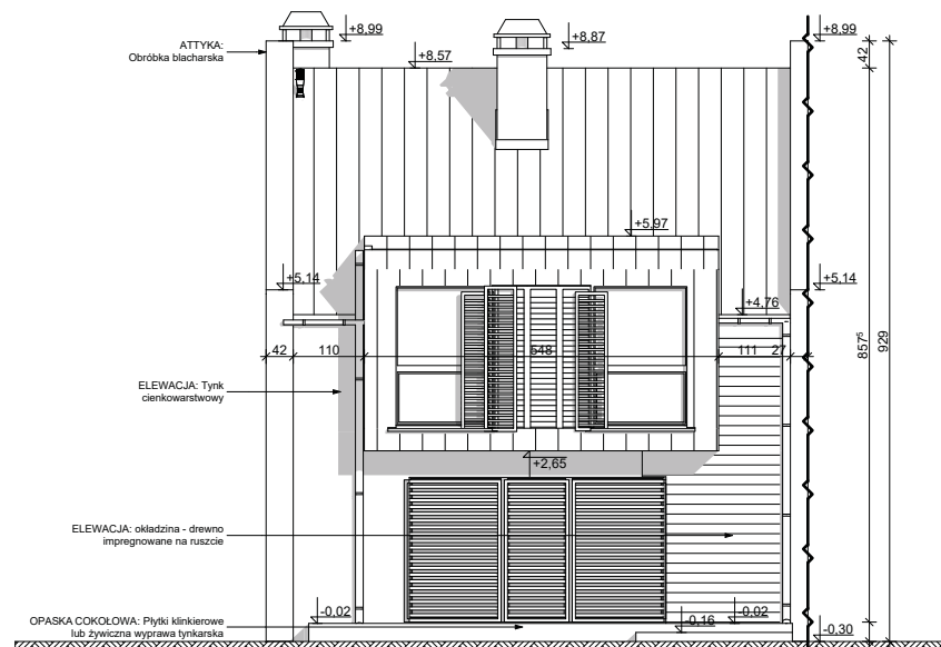
Elewacja tył
