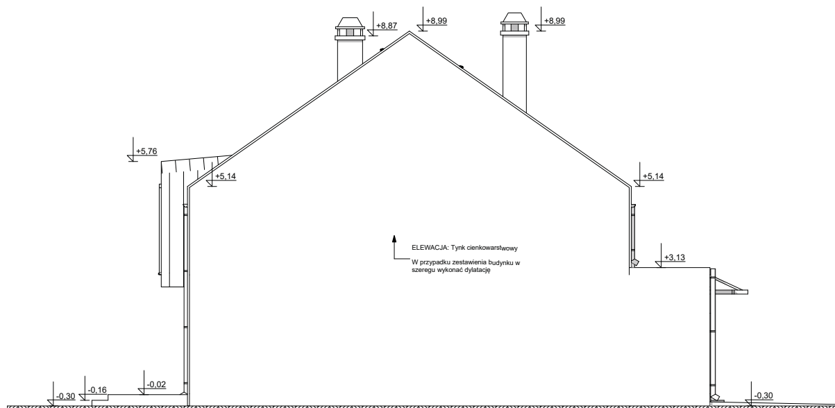
Elewacja bok
