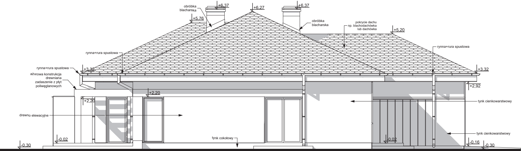
ELEWACJA BOCZNA
