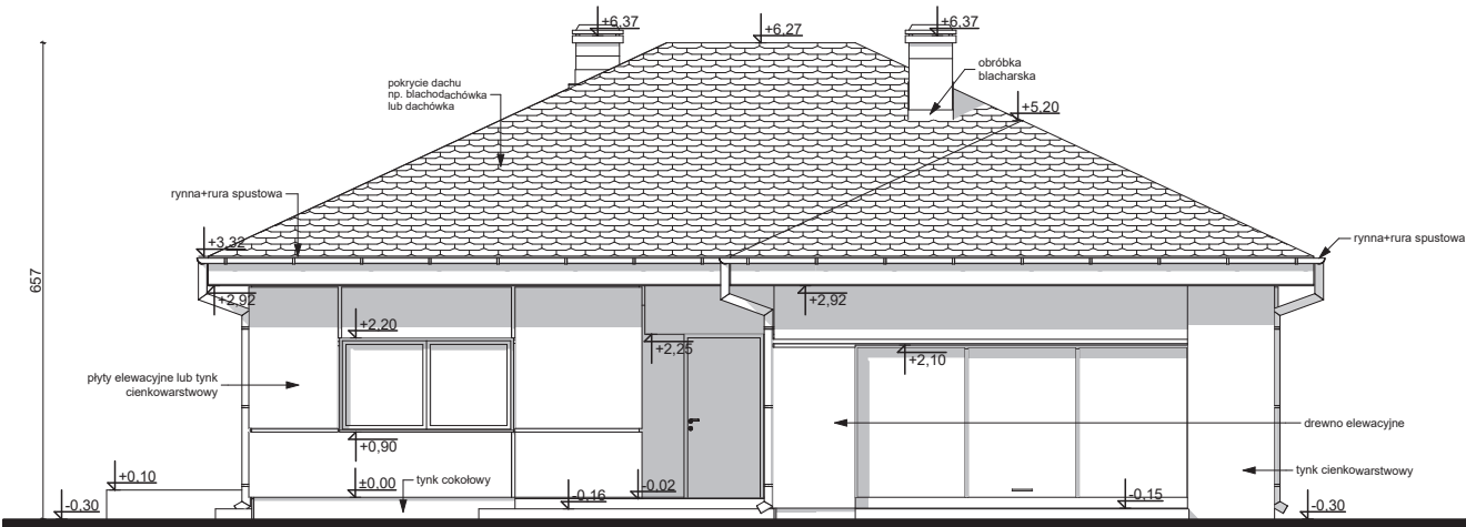
ELEWACJA FRONTOWA
