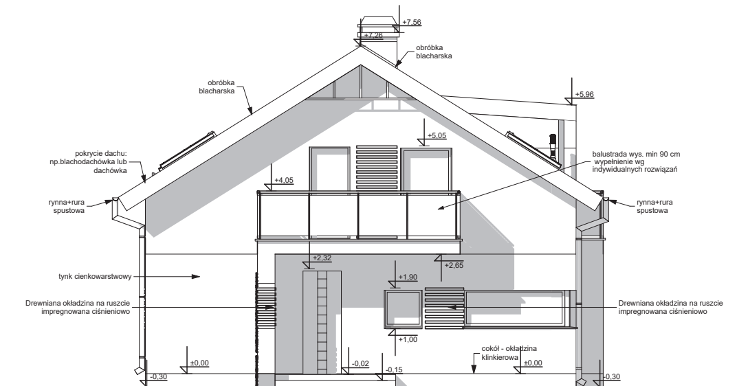
ELEWACJA FRONTOWA
