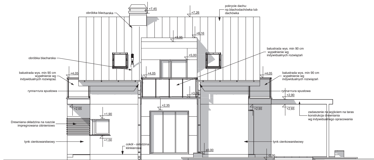
ELEWACJA BOCZNA
