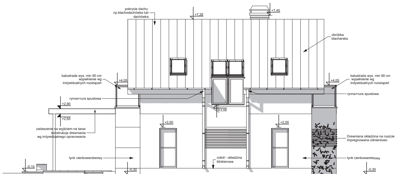
ELEWACJA BOCZNA
