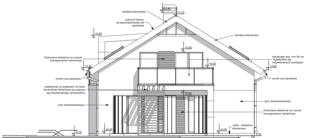
ELEWACJA TYLNA
