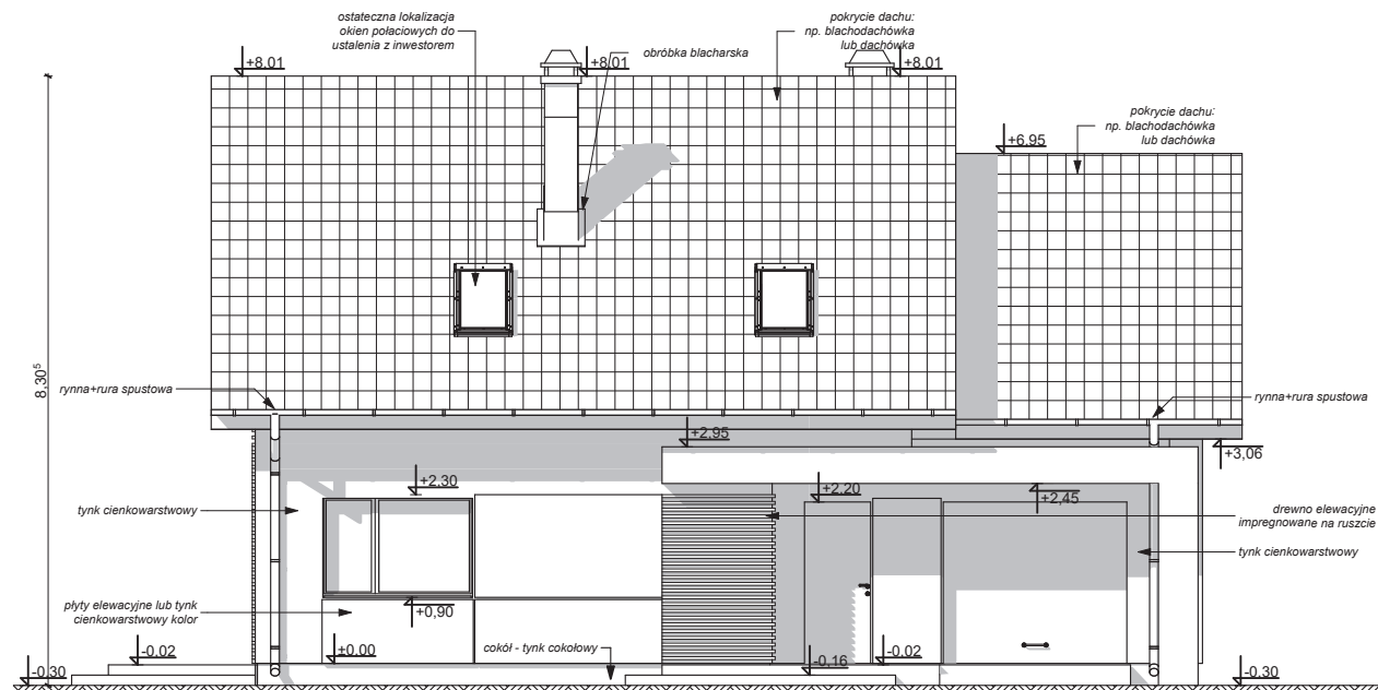
ELEWACJA FRONTOWA
