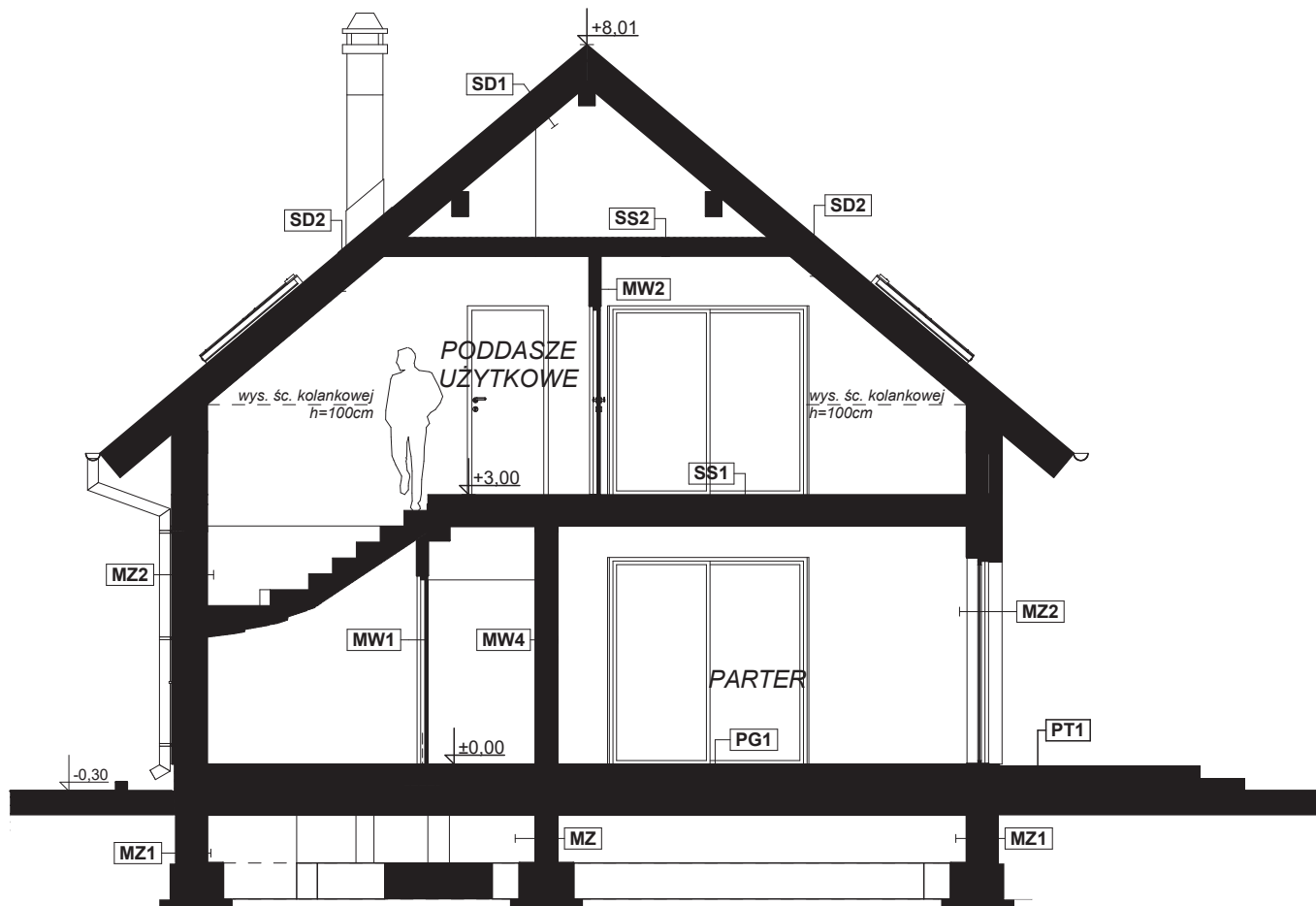
PRZEKRÓJ B-B
