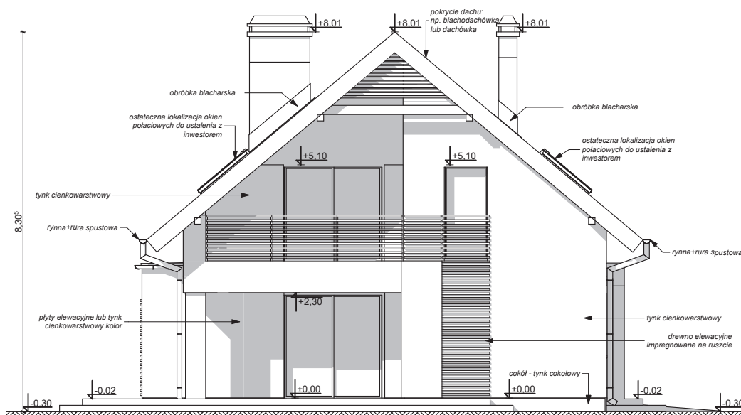
ELEWACJA BOCZNA
