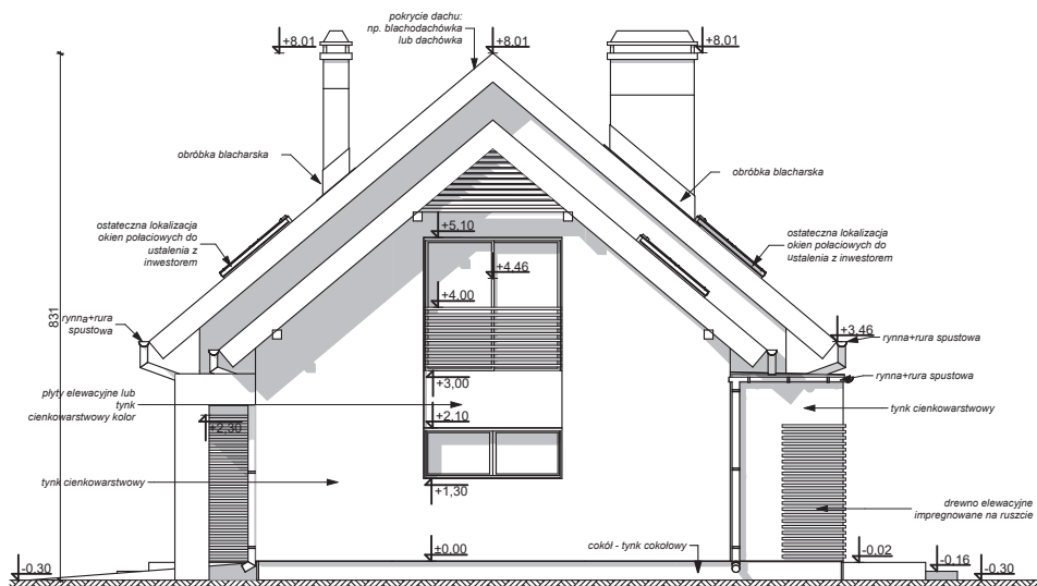
ELEWACJA BOCZNA
