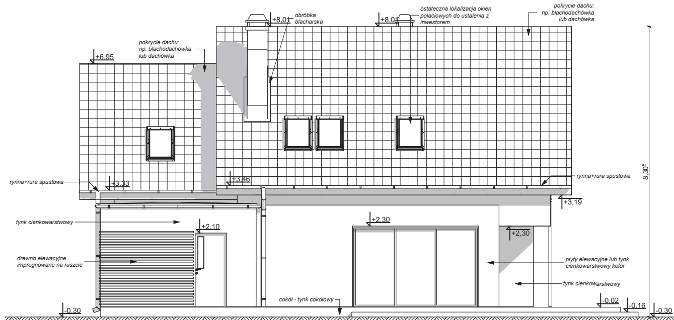
ELEWACJA TYLNA
