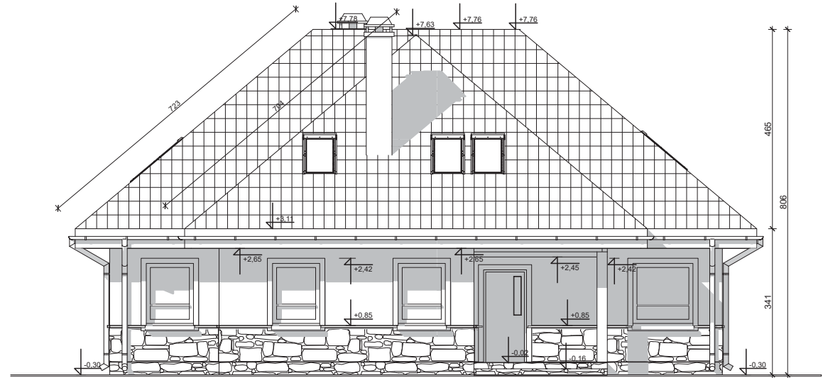
ELEWACJA FRONTOWA
