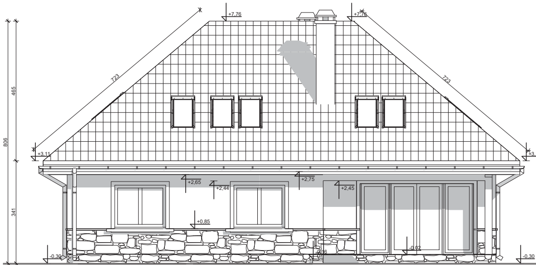
ELEWACJA TYLNA
