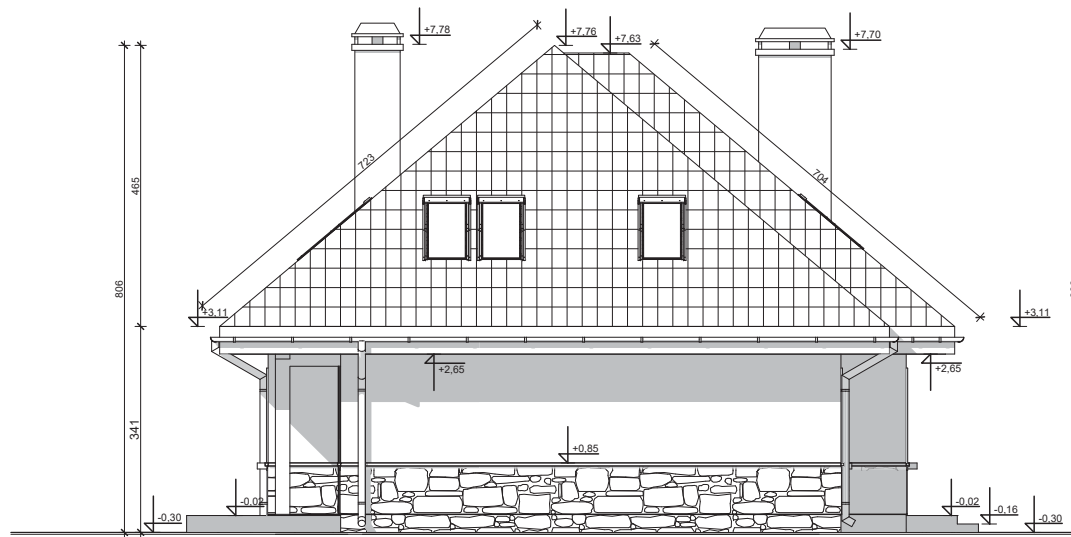
ELEWACJA BOCZNA
