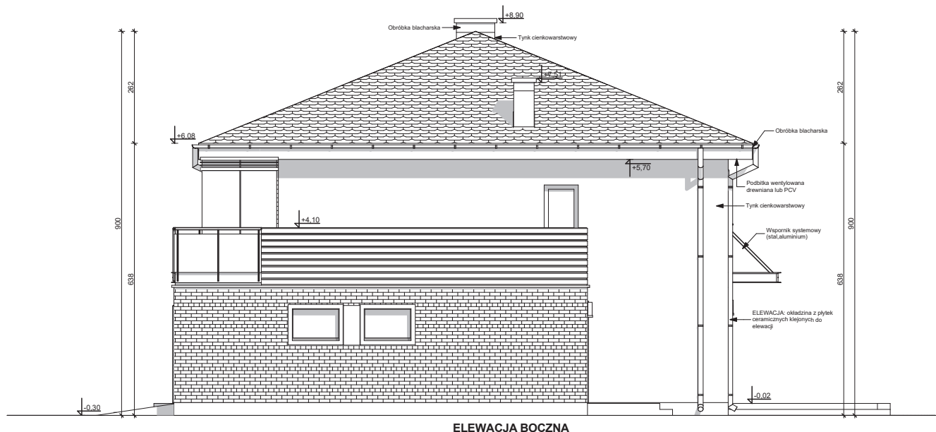
ELEWACJA BOCZNA
