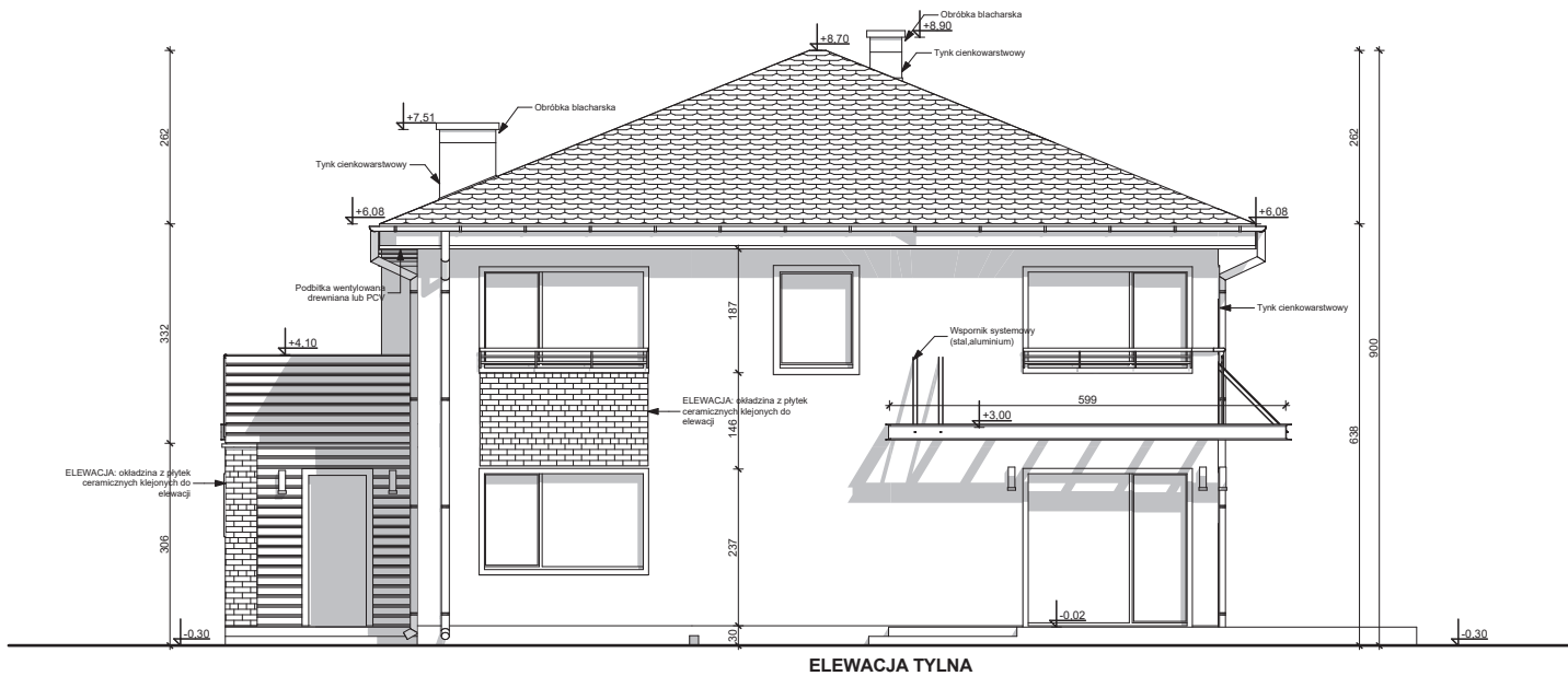
ELEWACJA TYLNA
