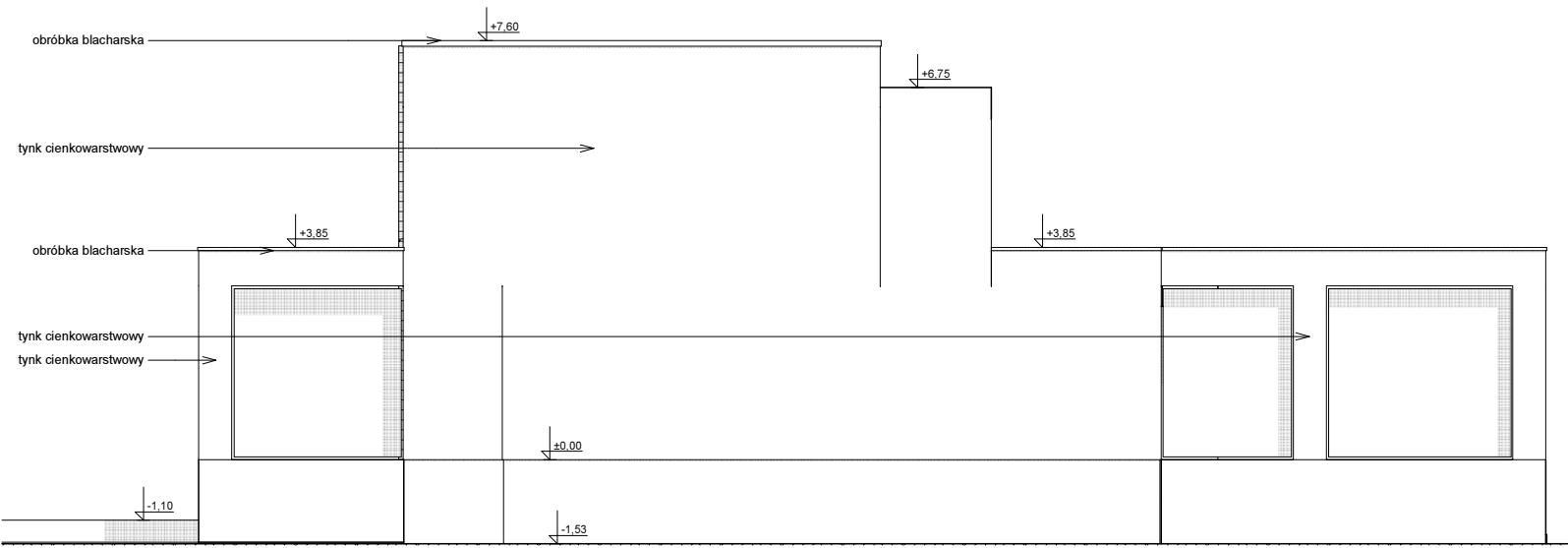
ELEWACJA BOCZNA
