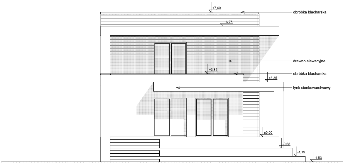
ELEWACJA TYLNA (ogrodowa)
