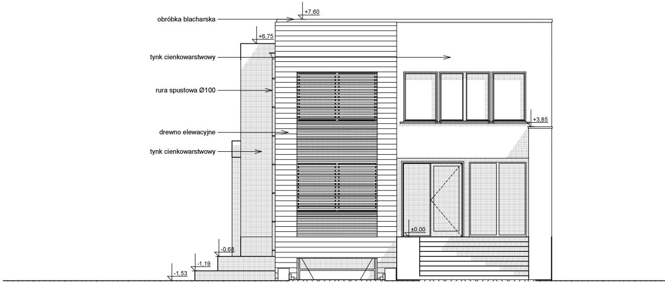
ELEWACJA FRONTOWA
