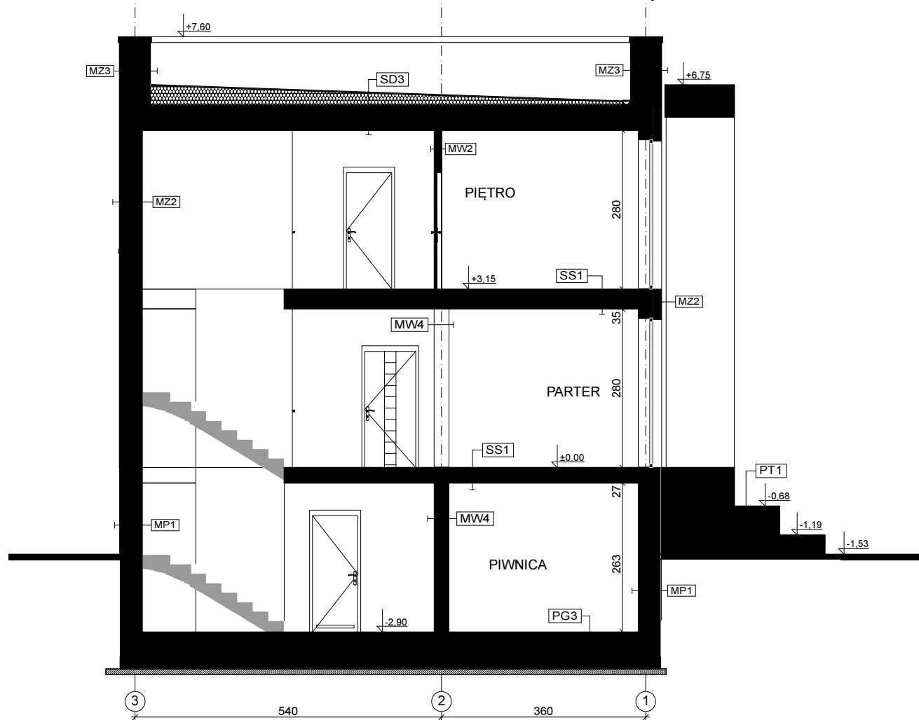
MZ2 - ŚCIANA ZEWN. KONSTR. OCIEPLONA
