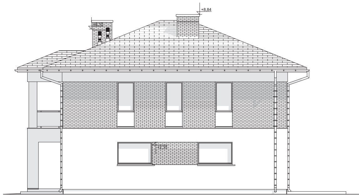
ELEWACJA BOCZNA
