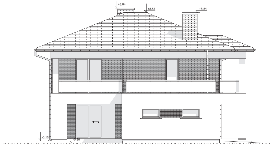
ELEWACJA BOCZNA
