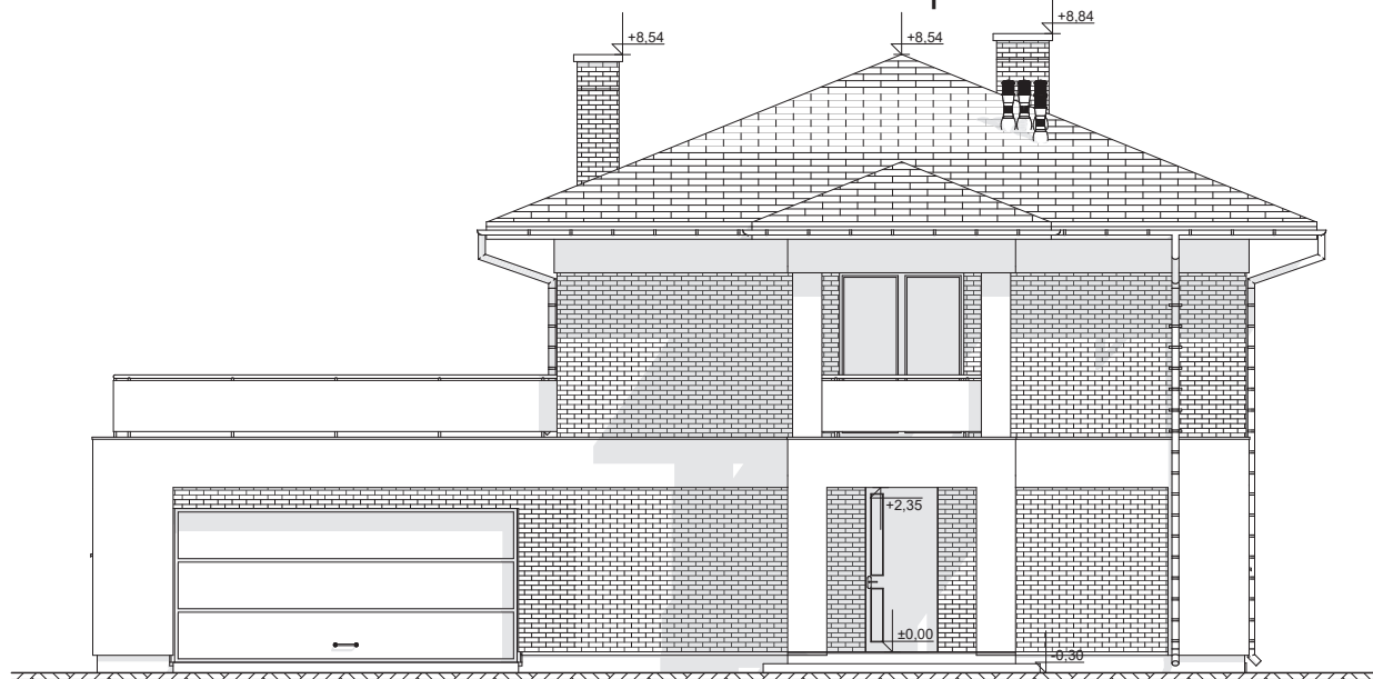
ELEWACJA FRONTOWA
