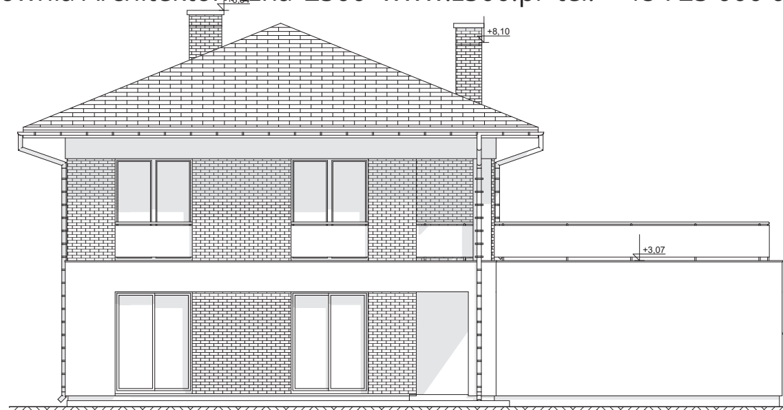
ELEWACJA OGRODOWA
