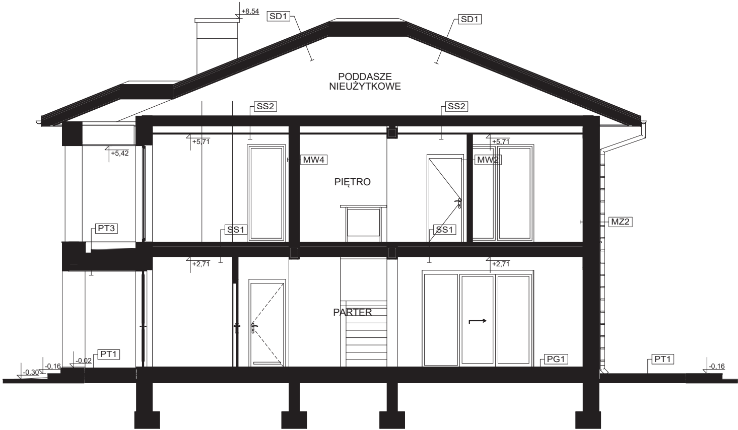
PRZEKRÓJ A-A
