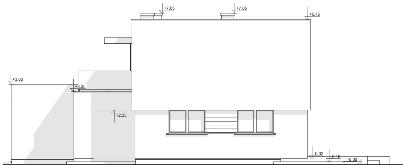
ELEWACJA BOCZNA
