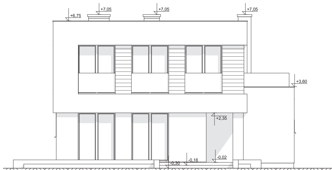
ELEWACJA OGRODOWA
