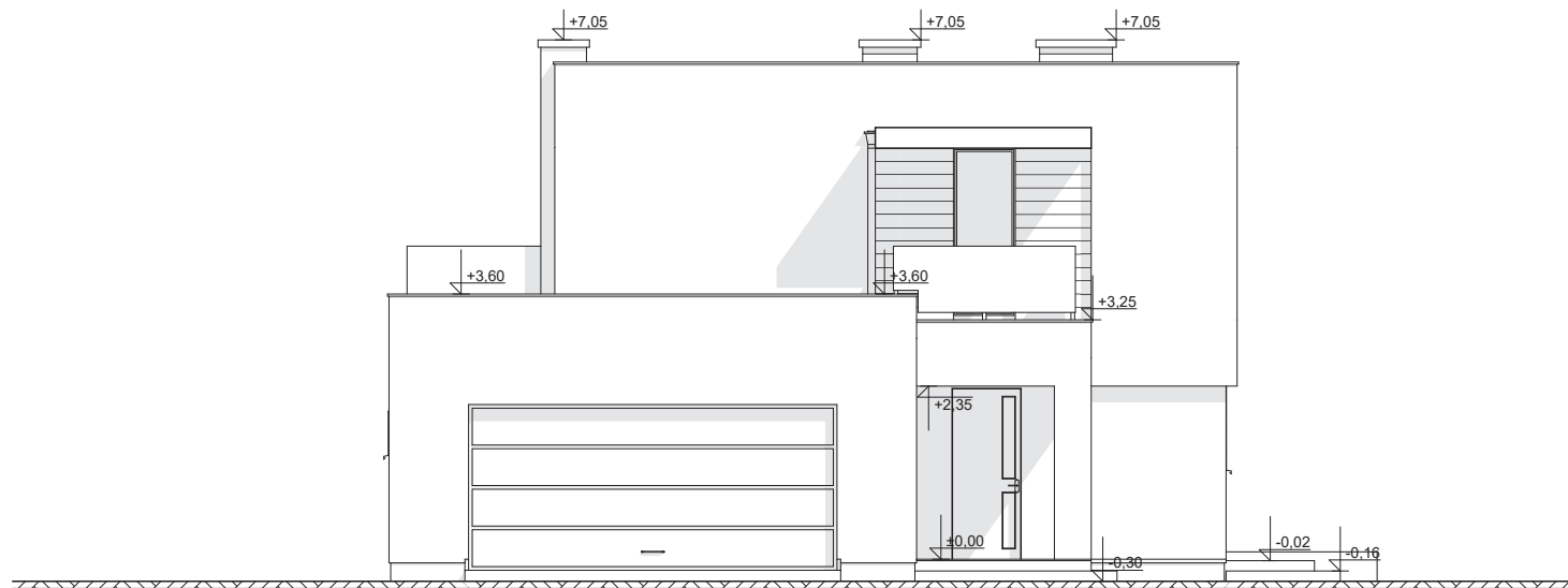
ELEWACJA FRONTOWA
