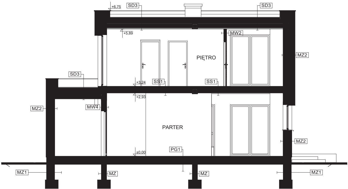
PRZEKRÓJ B-B
