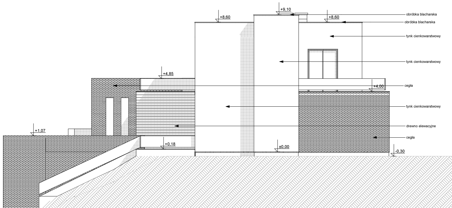
ELEWACJA BOCZNA
