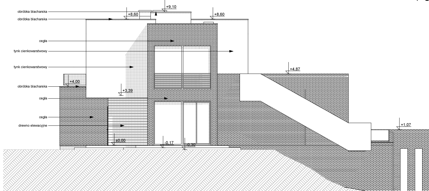
ELEWACJA BOCZNA
