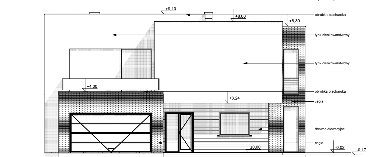
ELEWACJA FRONTOWA
