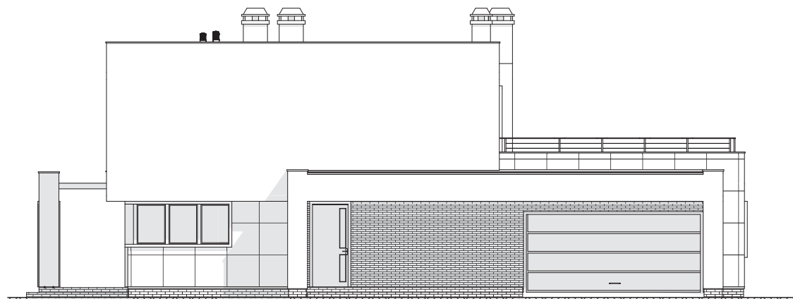
ELEWACJA FRONTOWA
