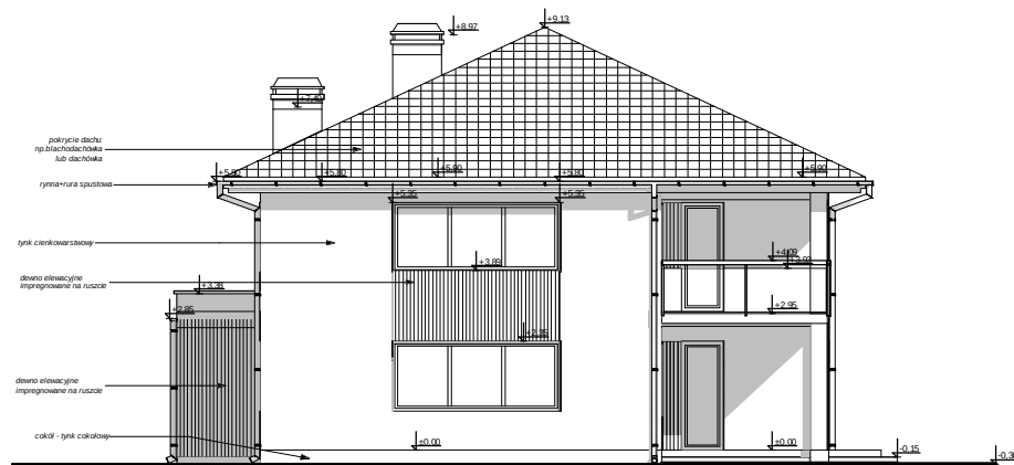
ELEWACJA OGRODOWA (tylna)
