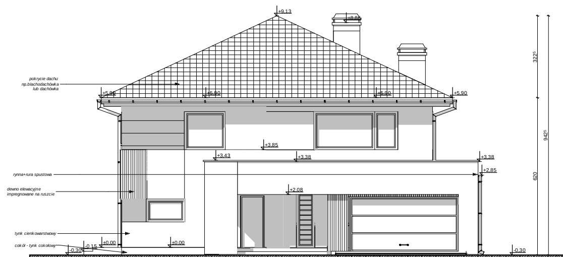
ELEWACJA FRONTOWA
