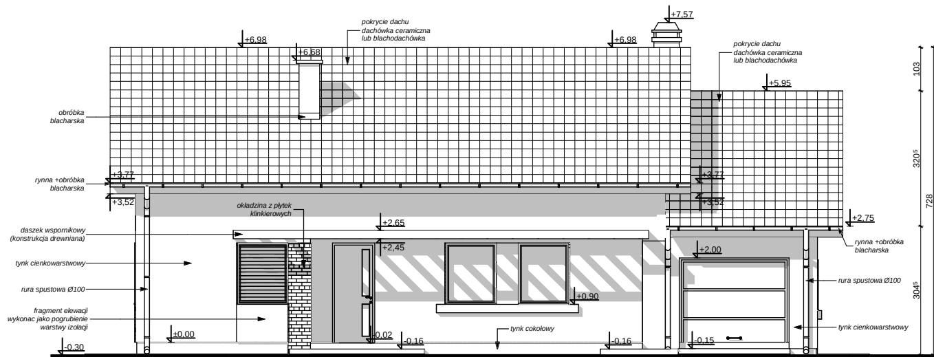
ELEWACJA FRONTOWA
