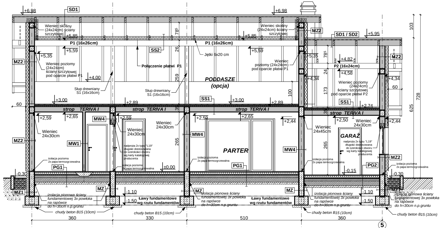
PRZEKRÓJ A-A
