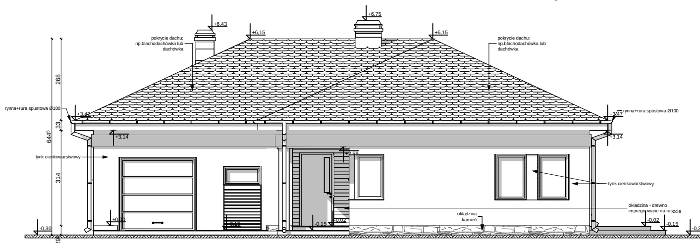
ELEWACJA FRONTOWA
