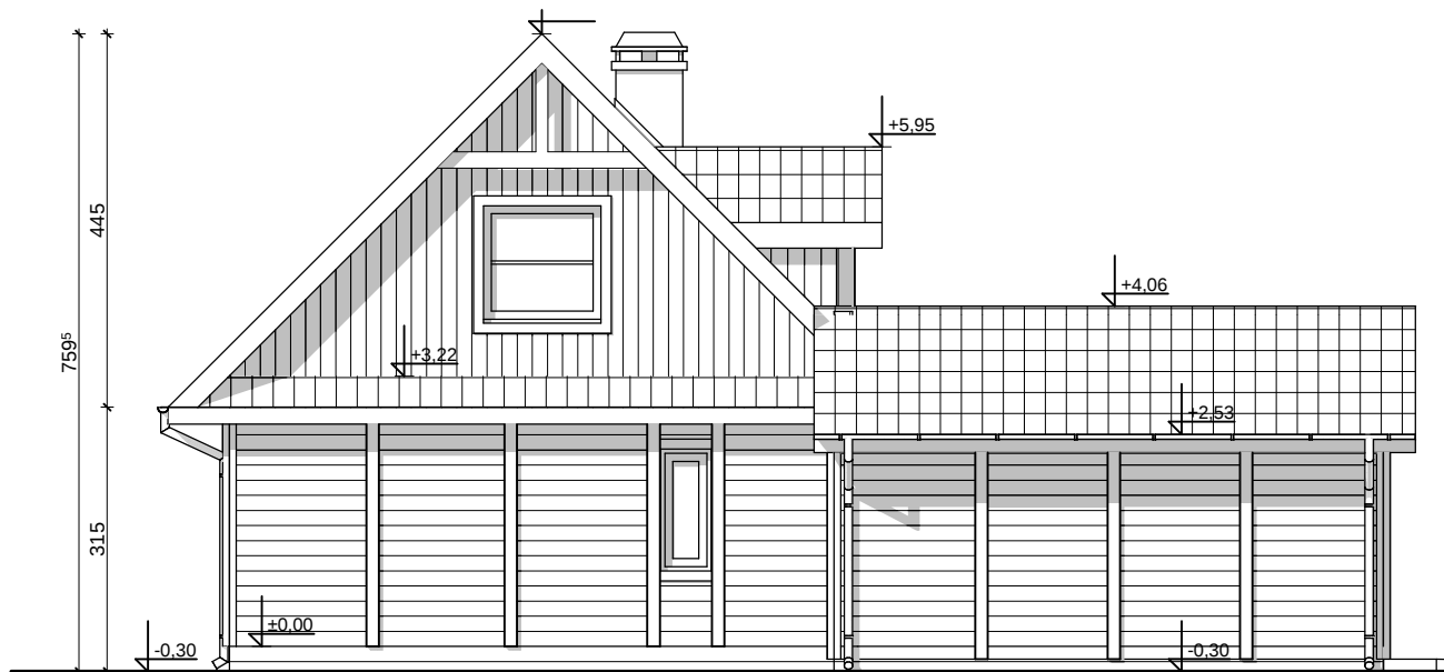
ELEWACJA BOCZNA
