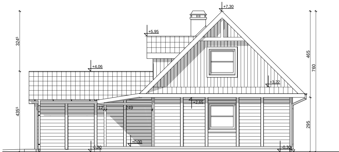
ELEWACJA BOCZNA
