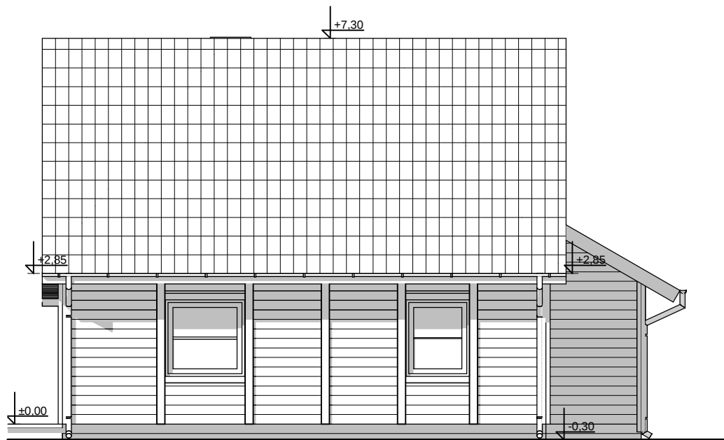
ELEWACJA OGRODOWA
