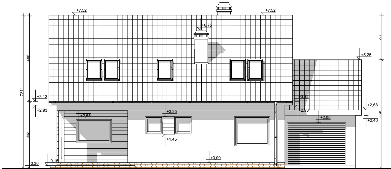
ELEWACJA FRONTOWA
