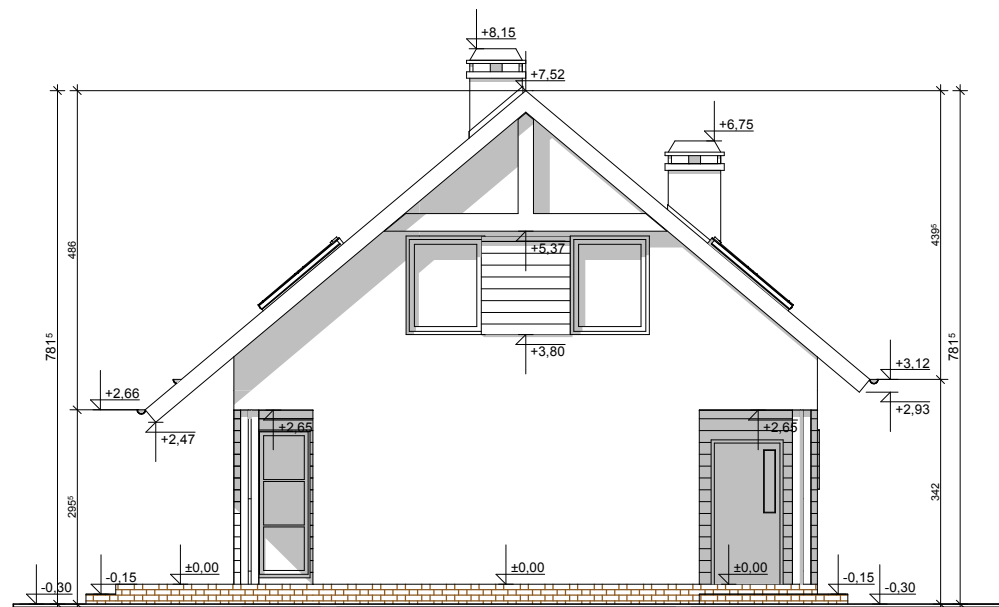
ELEWACJA BOCZNA
