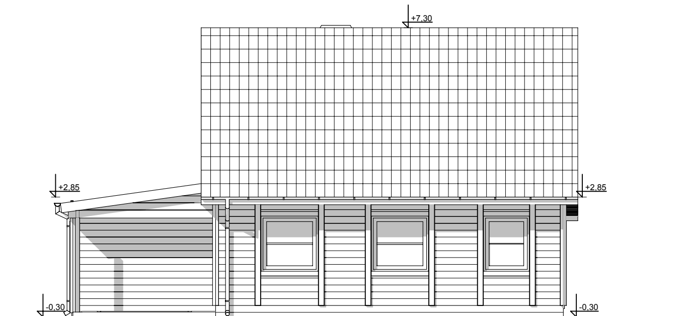
ELEWACJA OGRODOWA
