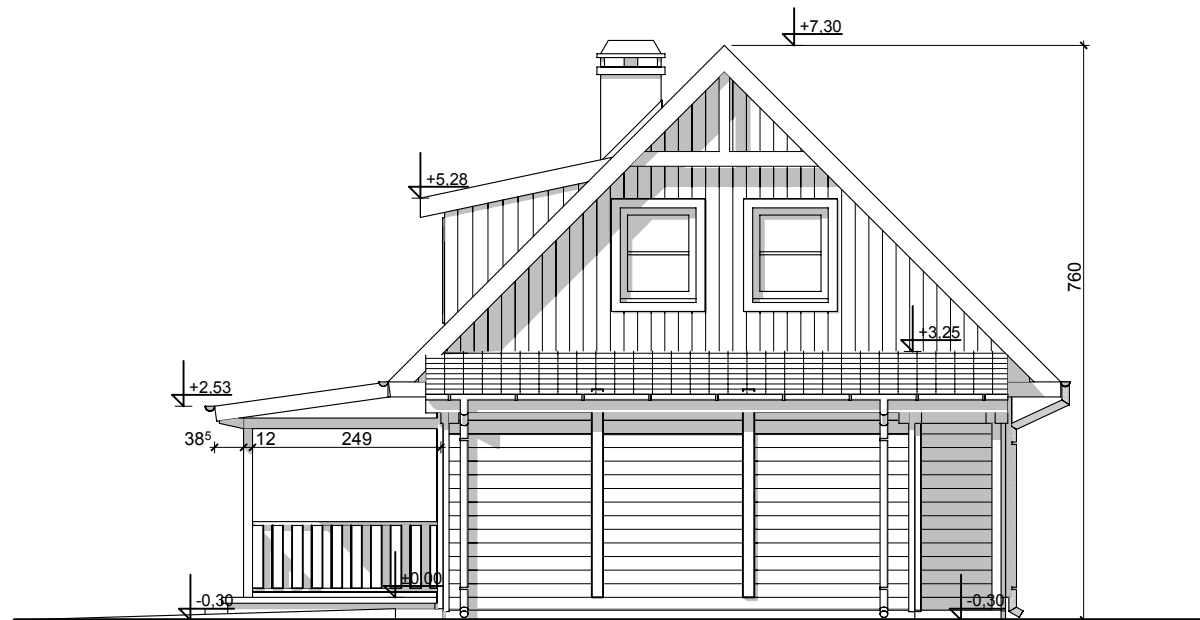
ELEWACJA BOCZNA
