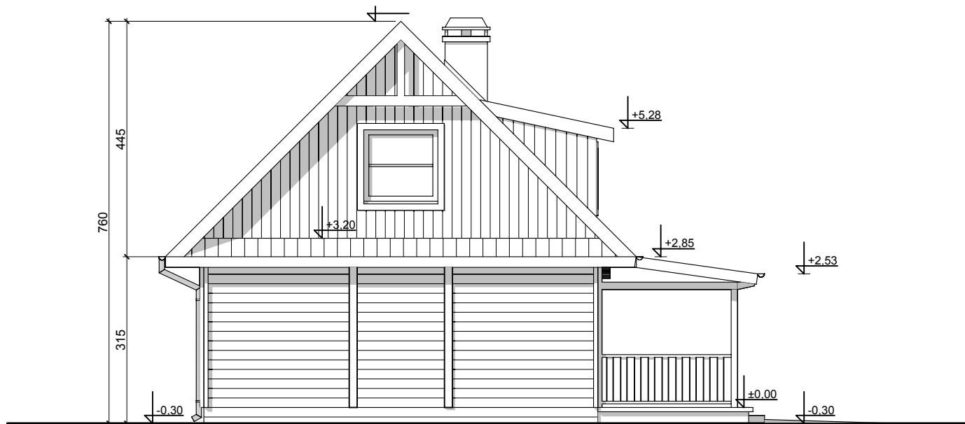
ELEWACJA BOCZNA
