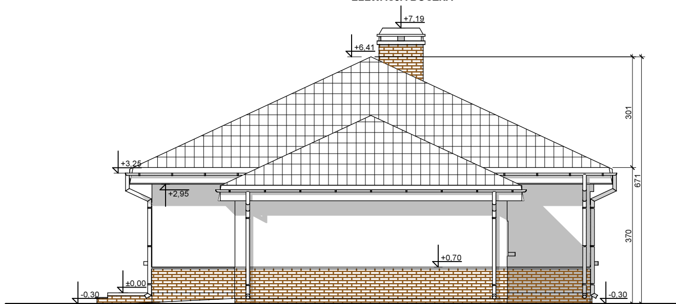
ELEWACJA BOCZNA
