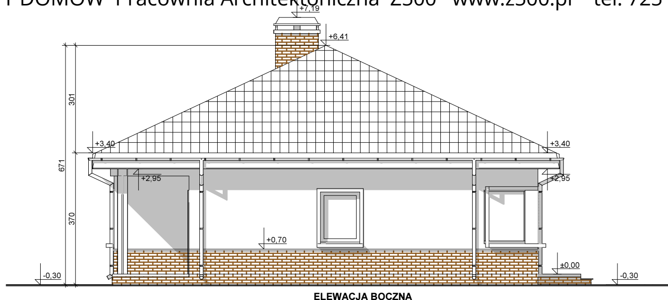
ELEWACJA BOCZNA
