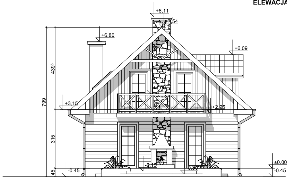
ELEWACJA FRONTOWA
