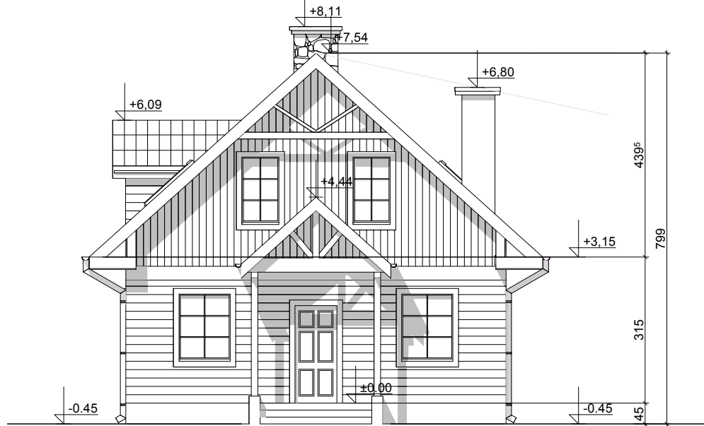
ELEWACJA FRONTOWA
