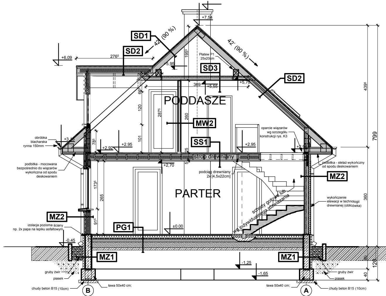
PRZEKRÓJ A-A
