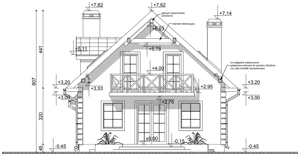
ELEWACJA TYLNA
