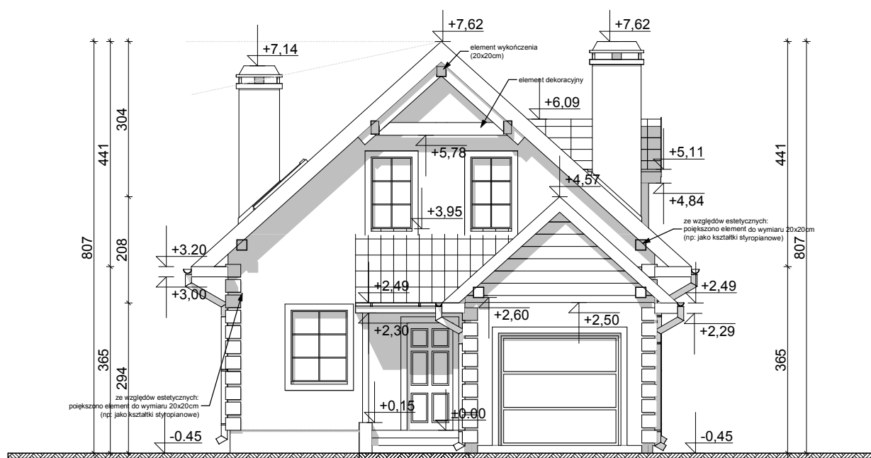
ELEWACJA FRONTOWA
