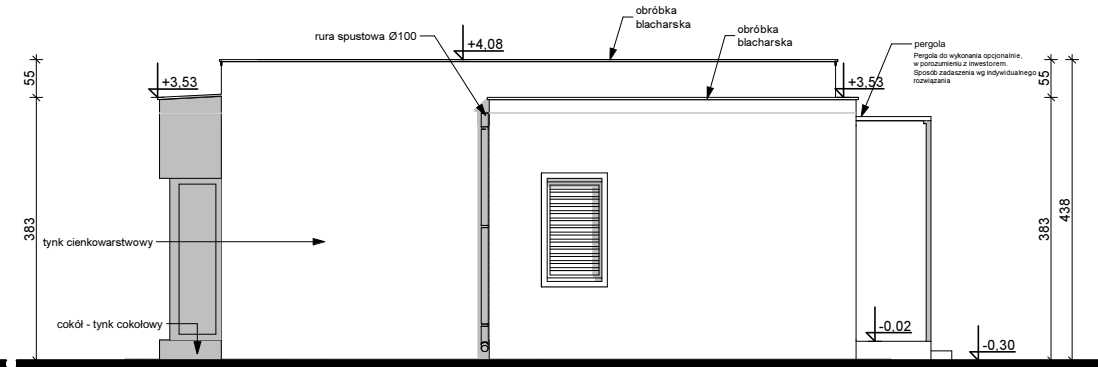
ELEWACJA TYLNA
