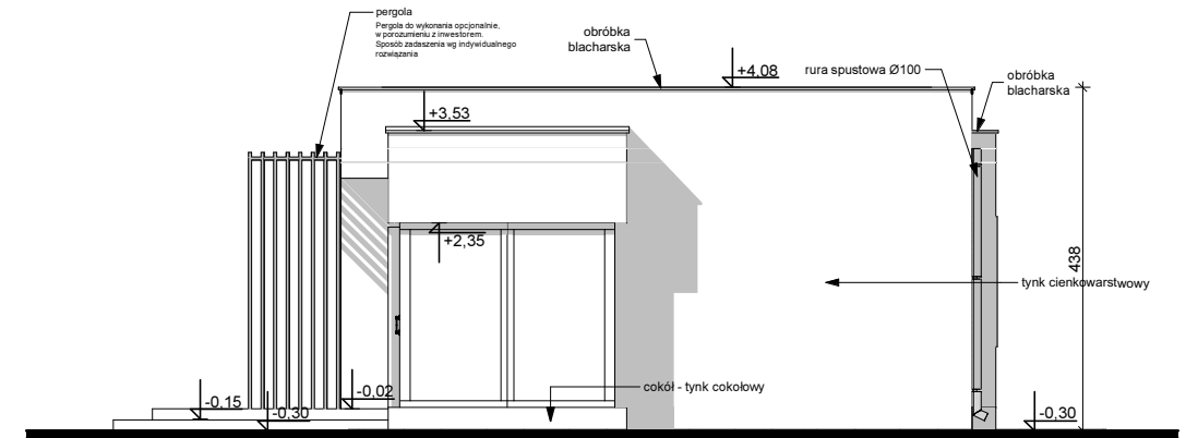
ELEWACJA TYLNA
