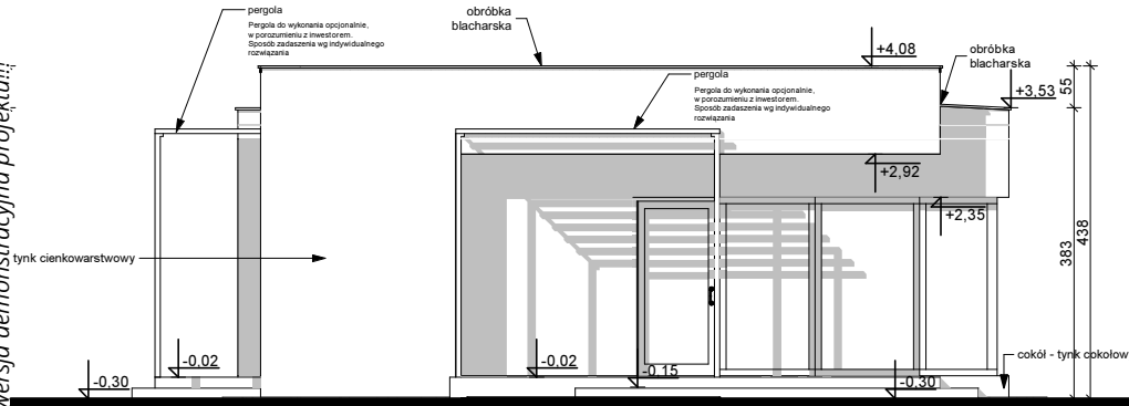
ELEWACJA FRONTOWA
