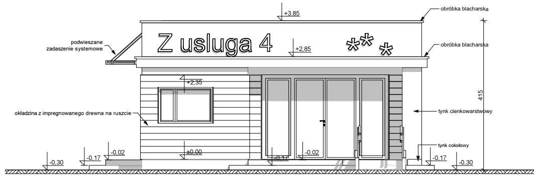
ELEWACJA FRONTOWA
