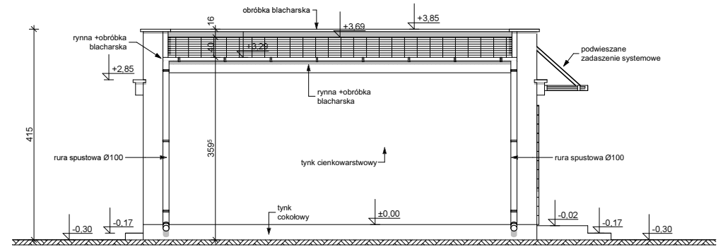
ELEWACJA TYLNA
