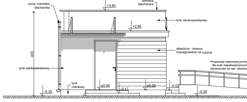
ELEWACJE BOCZNE
