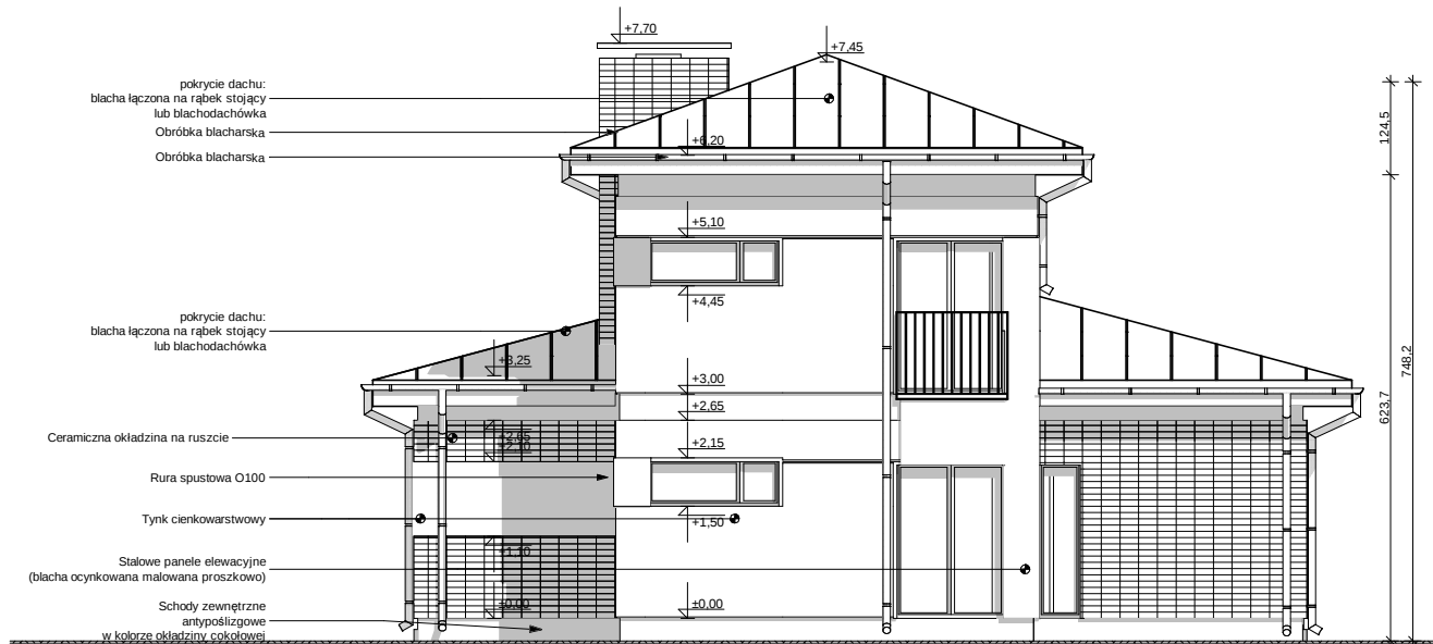
ELEWACJA OGRODOWA (tylna)
