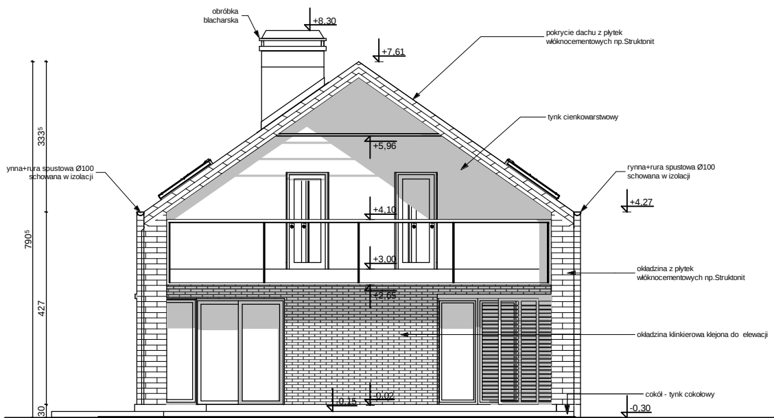
ELEWACJA ogrodowa
