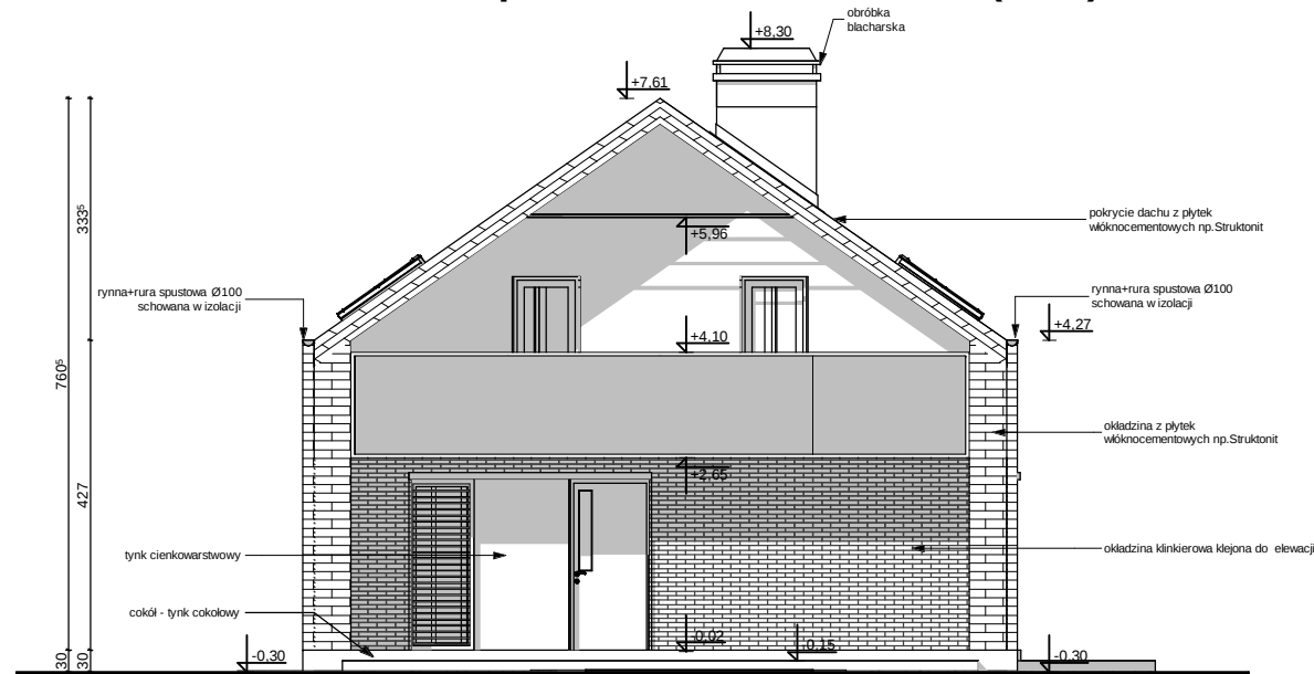
ELEWACJA FRONTOWA
