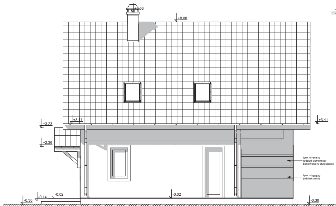
ELEWACJA BOCZNA
