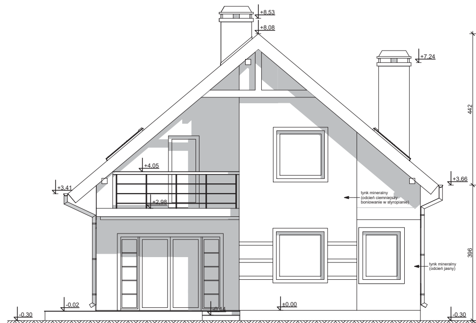
ELEWACJA OGRODOWA
