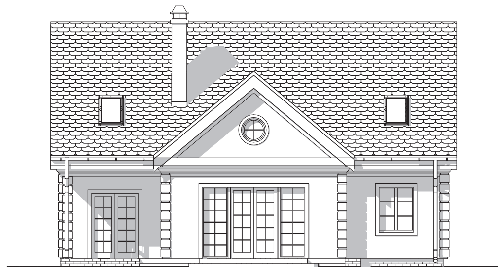
ELEWACJA OGRODOWA
