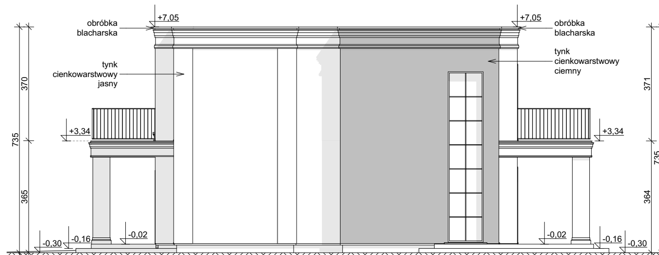
ELEWACJA BOCZNA
