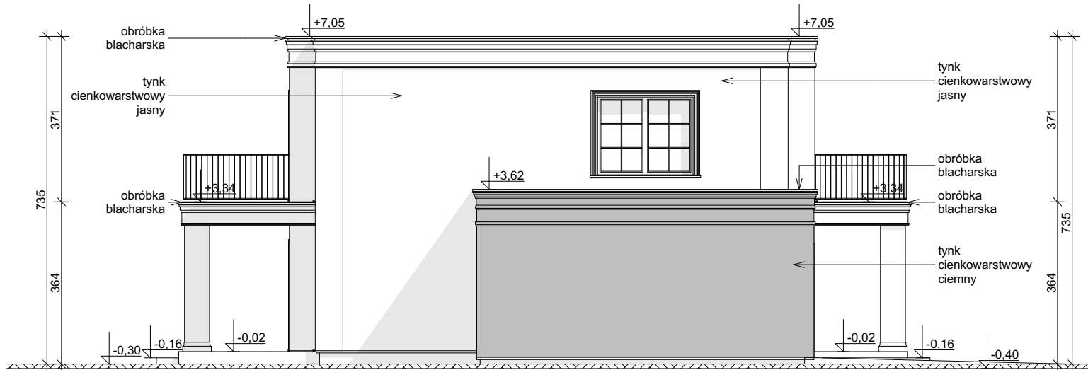
ELEWACJA BOCZNA
