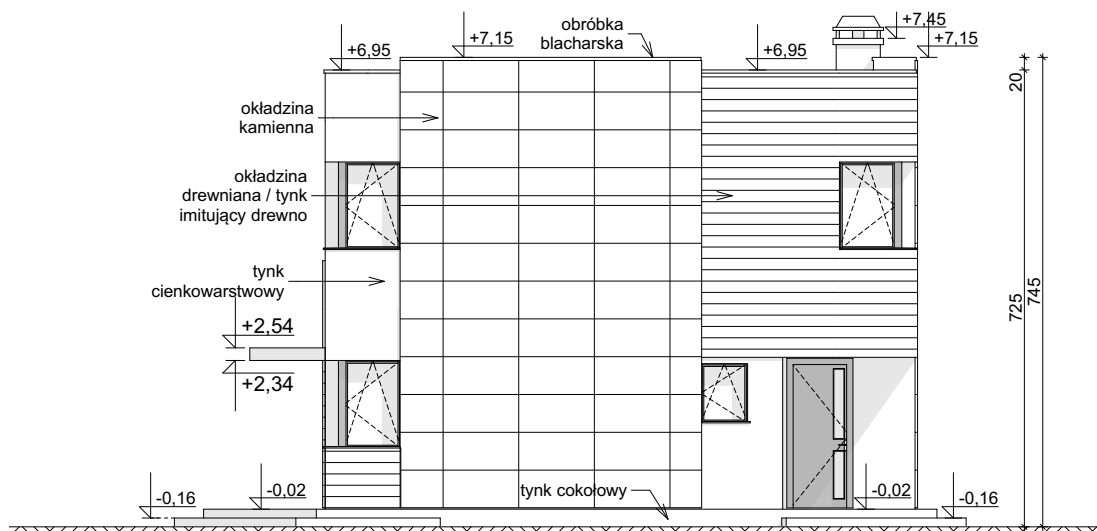
ELEWACJA BOCZNA
