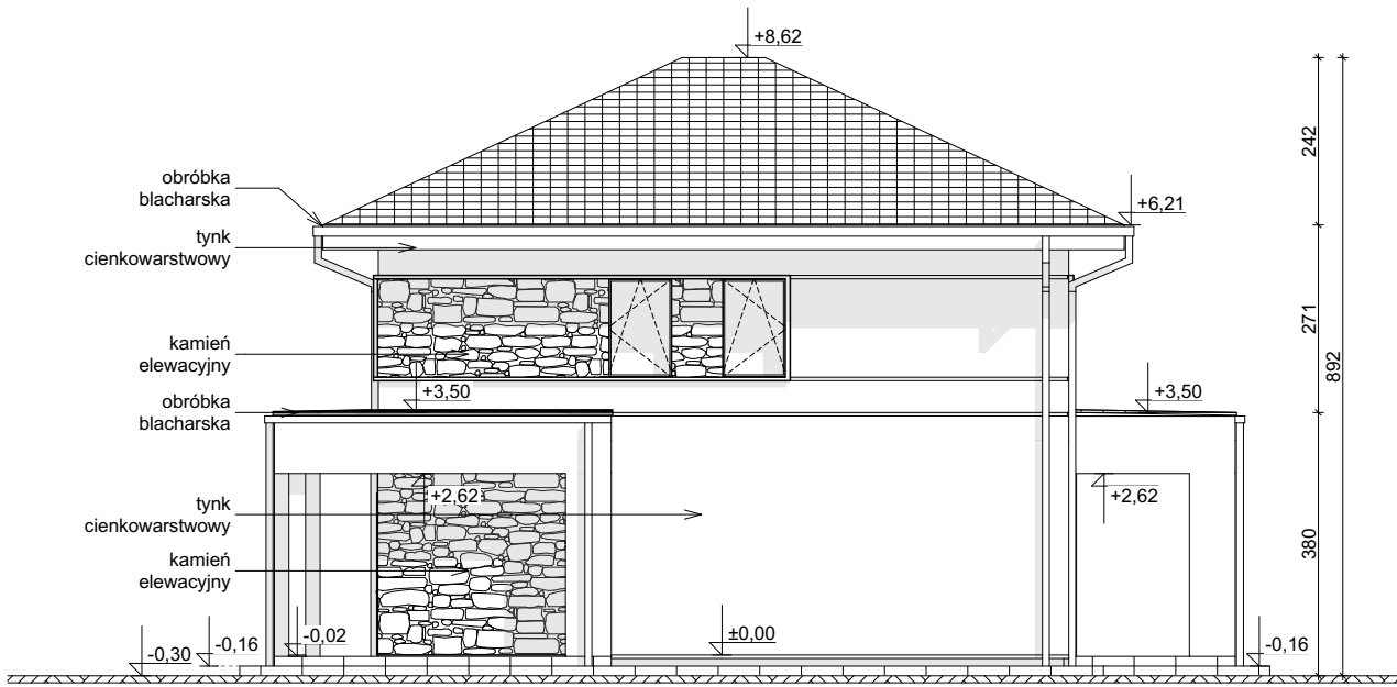
ELEWACJA BOCZNA
