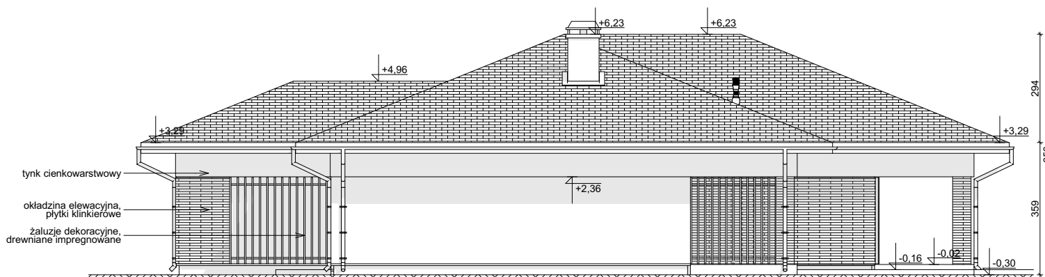
ELEWACJA BOCZNA
