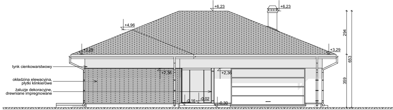
ELEWACJA FRONTOWA
