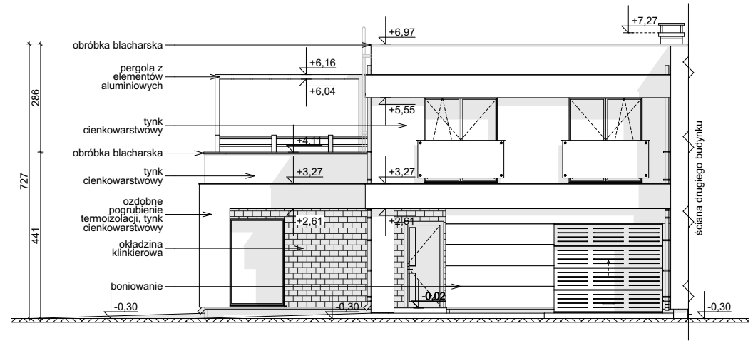
ELEWACJA FRONTOWA
