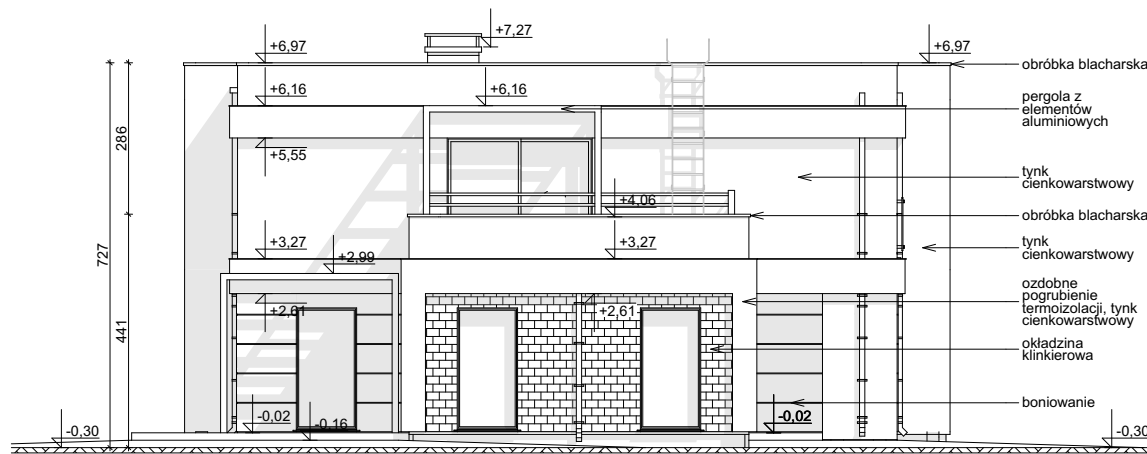
ELEWACJA BOCZNA
