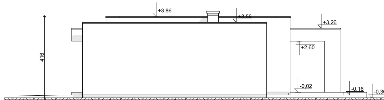
ELEVACJA BOCZNA
