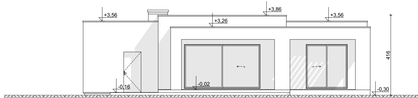
ELEVACJA OGRODOWA
