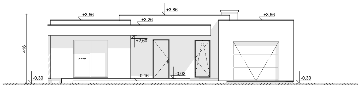
ELEWACJA FRONTOWA
