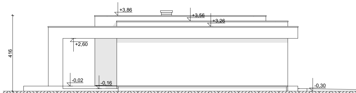
ELEWACJA BOCZNA
