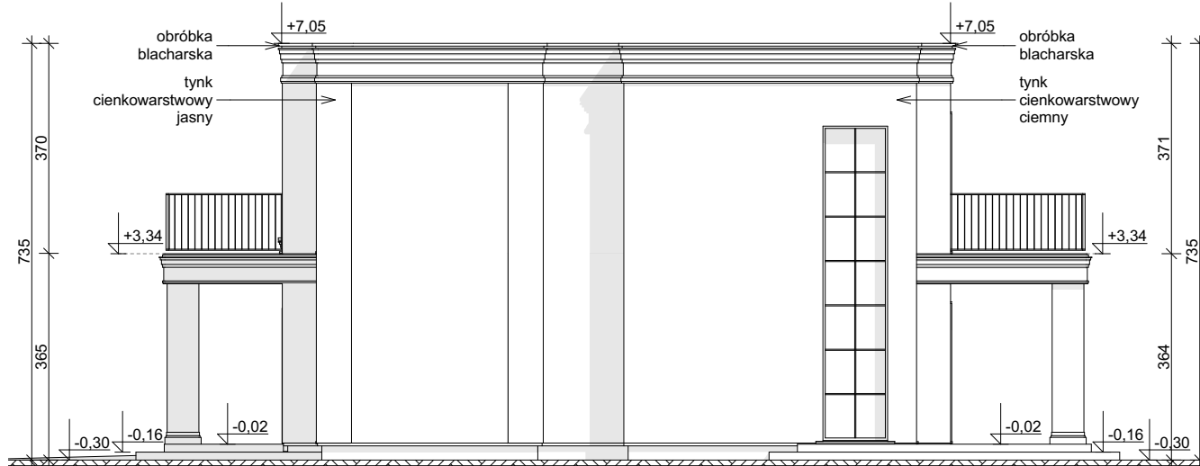
ELEWACJA BOCZNA
