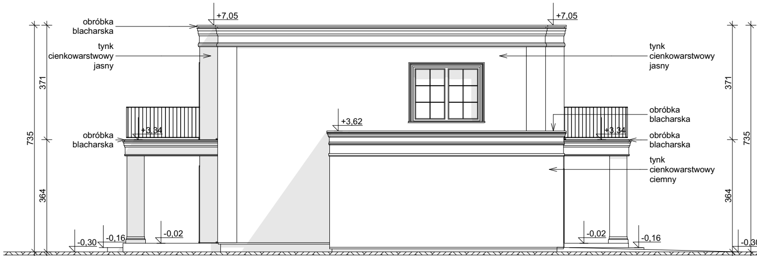
ELEWACJA BOCZNA
