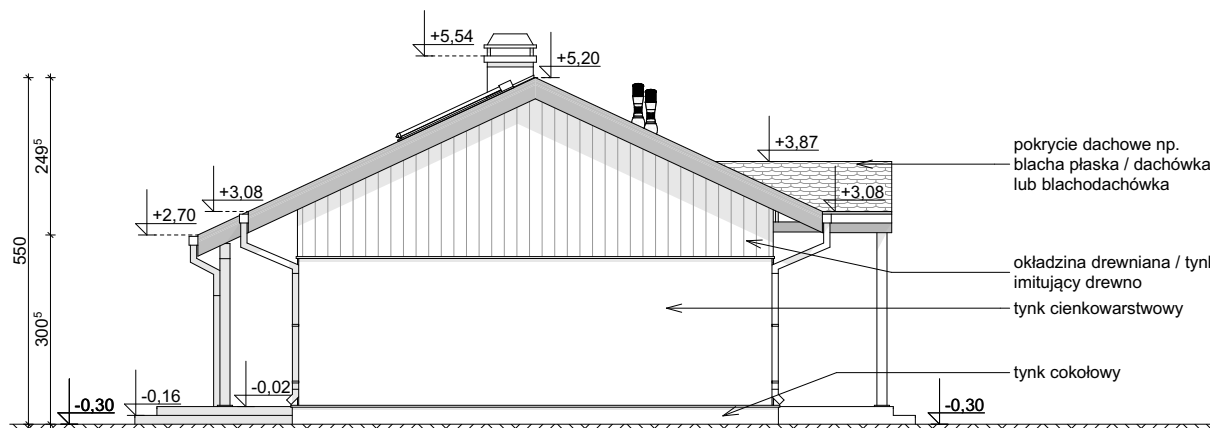
ELEWACJA BOCZNA
