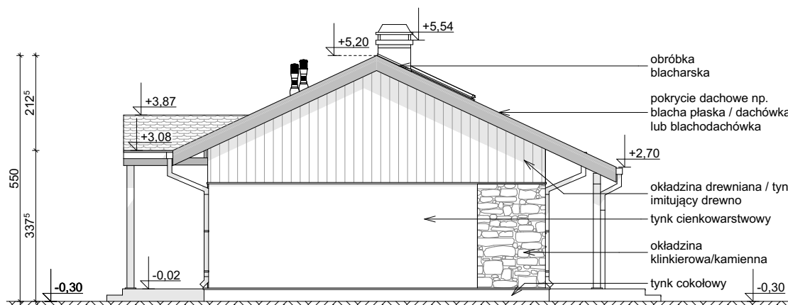
ELEWACJA BOCZNA
