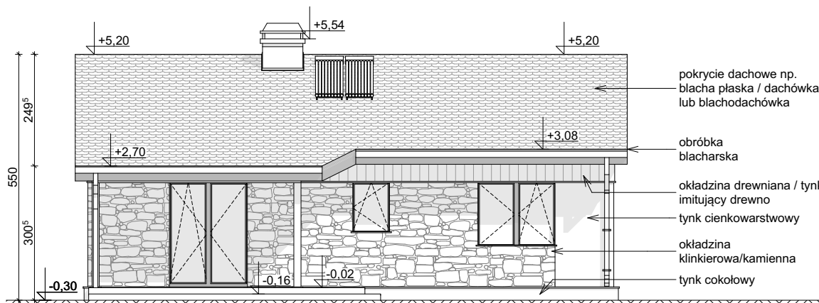
ELEWACJA OGRODOWA
