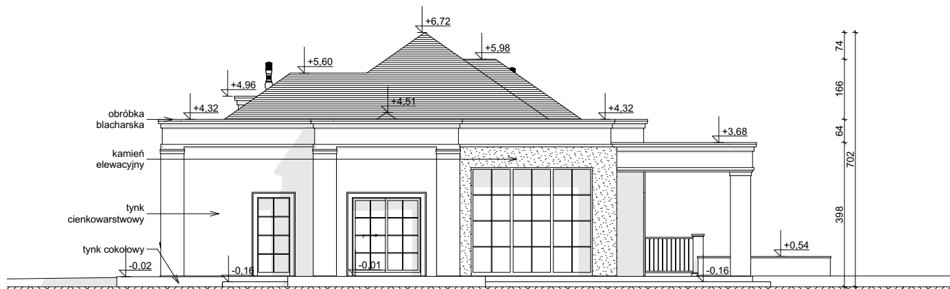
ELEWACJA BOCZNA
