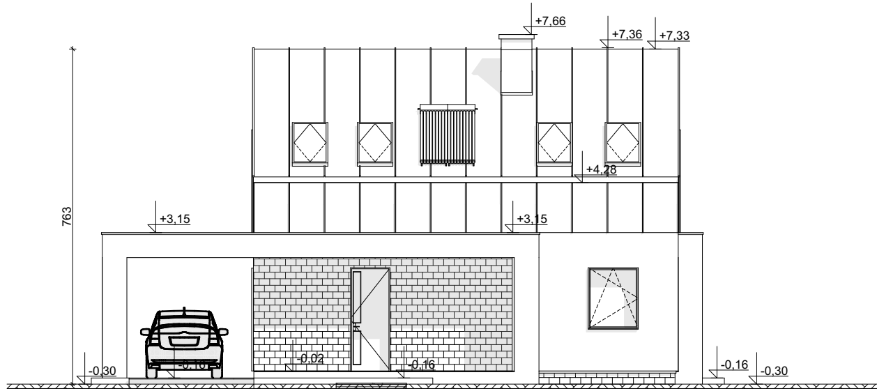
ELEWACJA FRONTOWA
