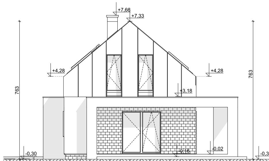
ELEVACJA BOCZNA
